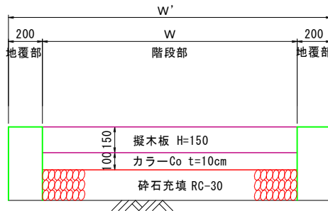
A-A' 断面図
