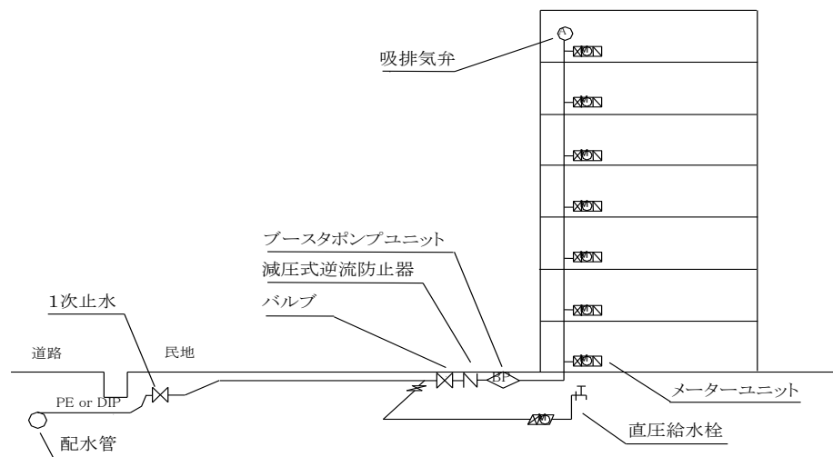
図 7-8 直結直圧と直結増圧の併用
