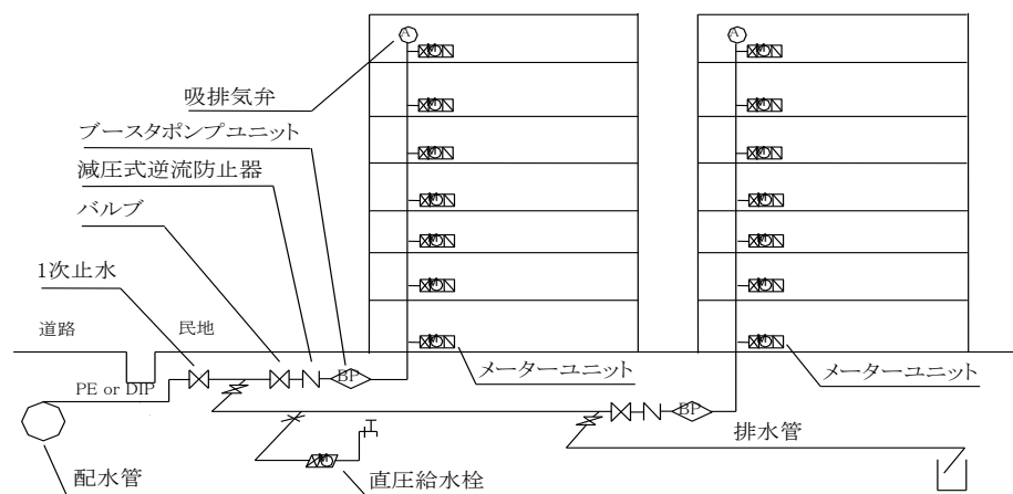
図 7-9 複数の建築物に直結増圧
