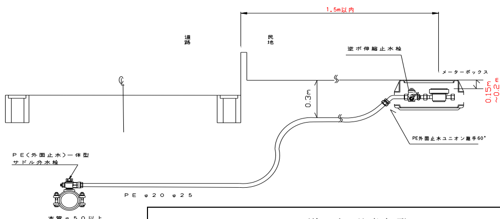
図 5-3 配水管 \phi 50\text{mm} 以上×給水管 \phi 20 \cdot \phi 25 の標準図
