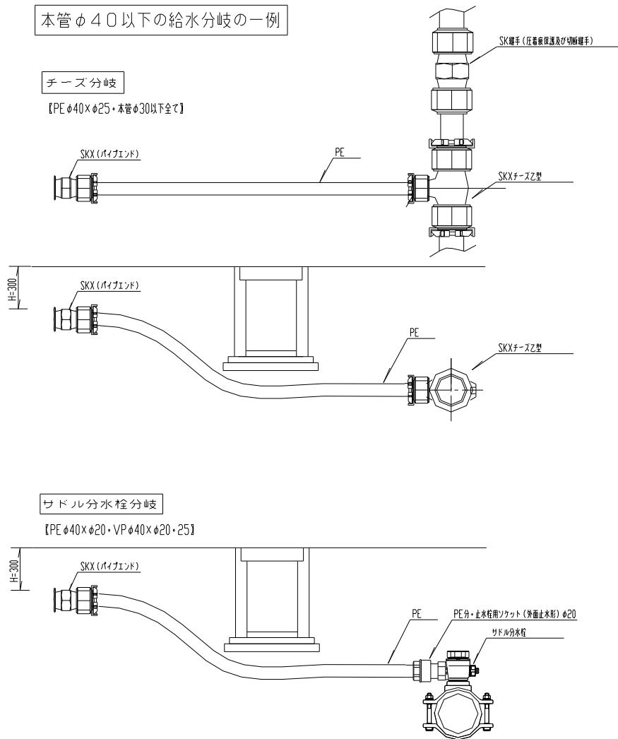
配水管 \phi 40\text{mm} 以下 \times 給水管 \phi 20 \cdot \phi 25 の標準図
