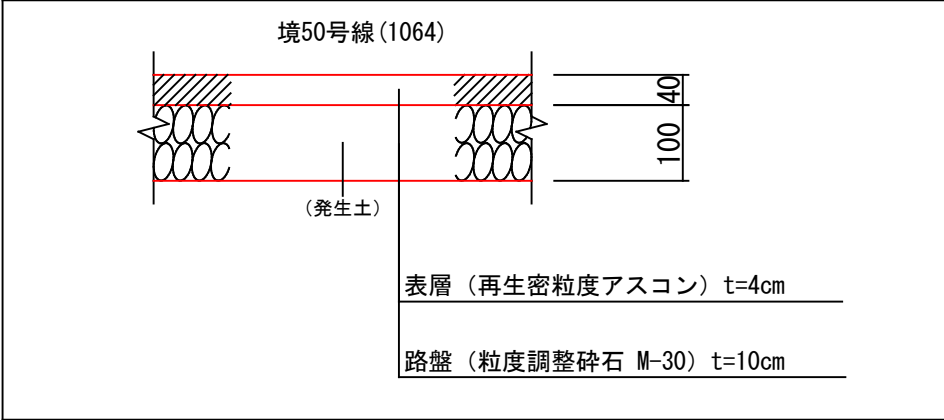
舗装復旧構成図 s=1:10
