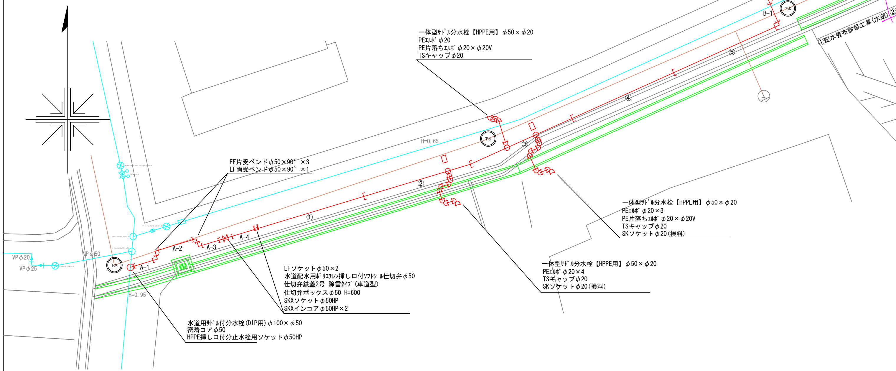
本設詳細図 S=1:100
