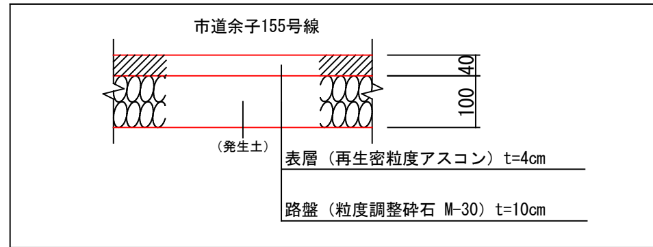
舗装復旧構成図 s=1:10
