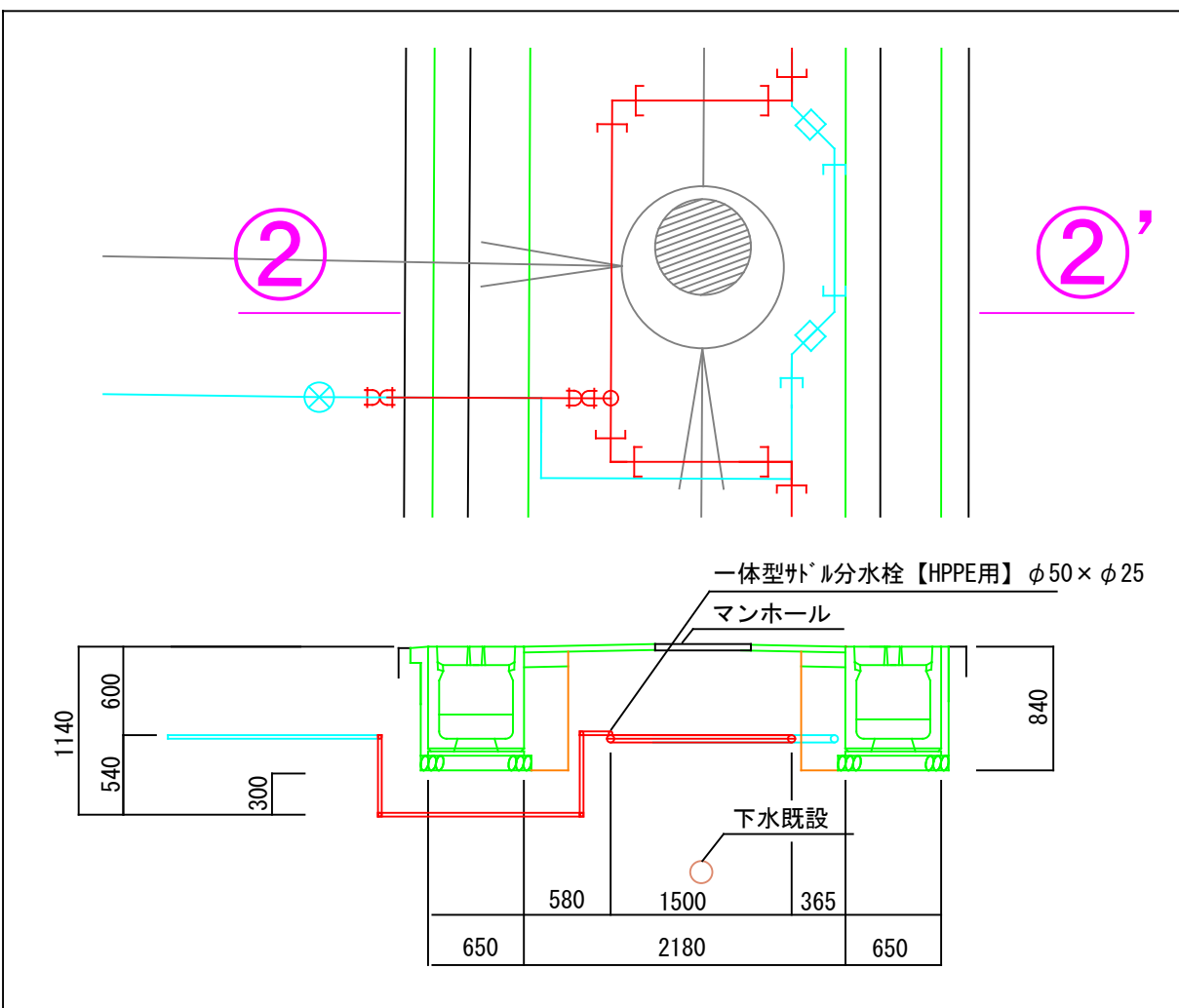
切廻し詳細図② s=1:50
