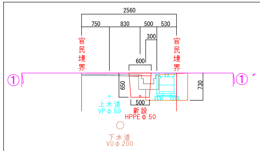
舗装復旧構成図 s=1:10
