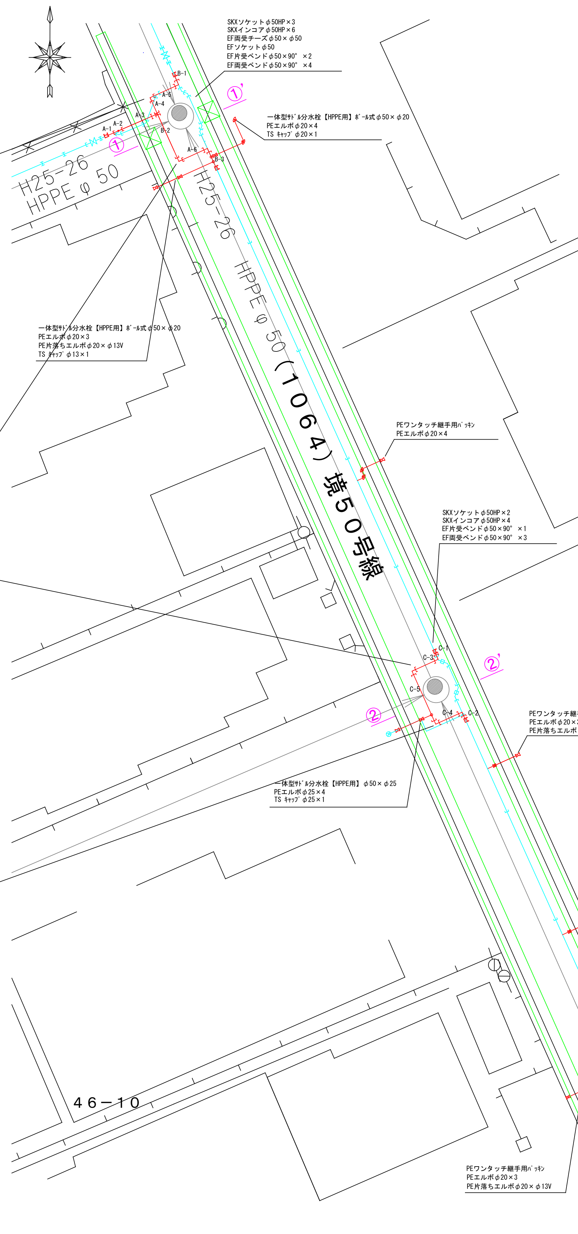
本設詳細図 S=1:100
