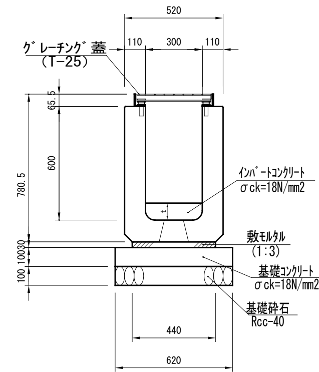
可変側溝 (4No.5付近)
