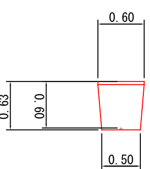
標準掘削断面図
