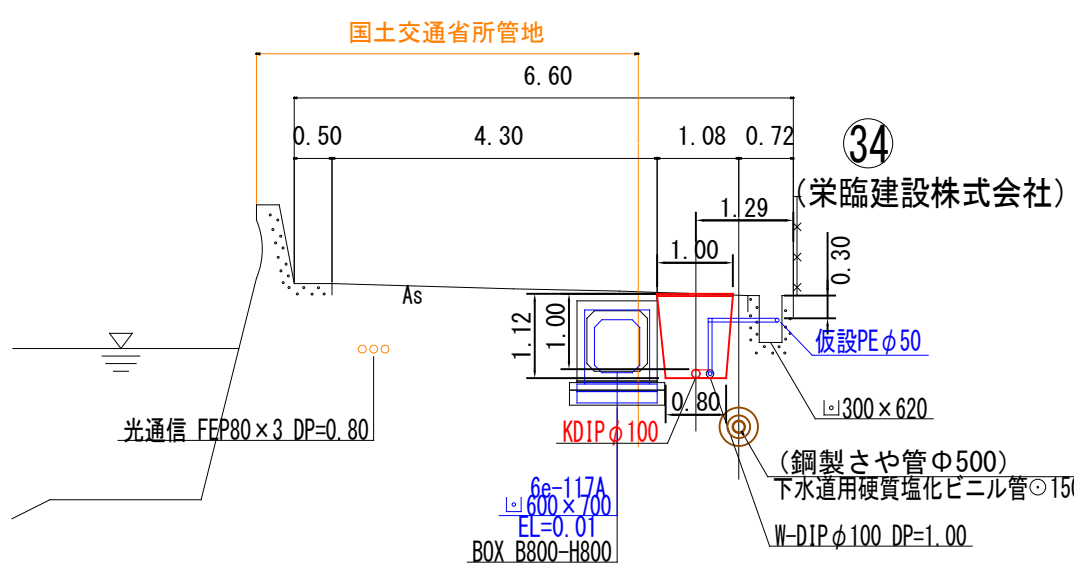
詳細図 S=1:100
