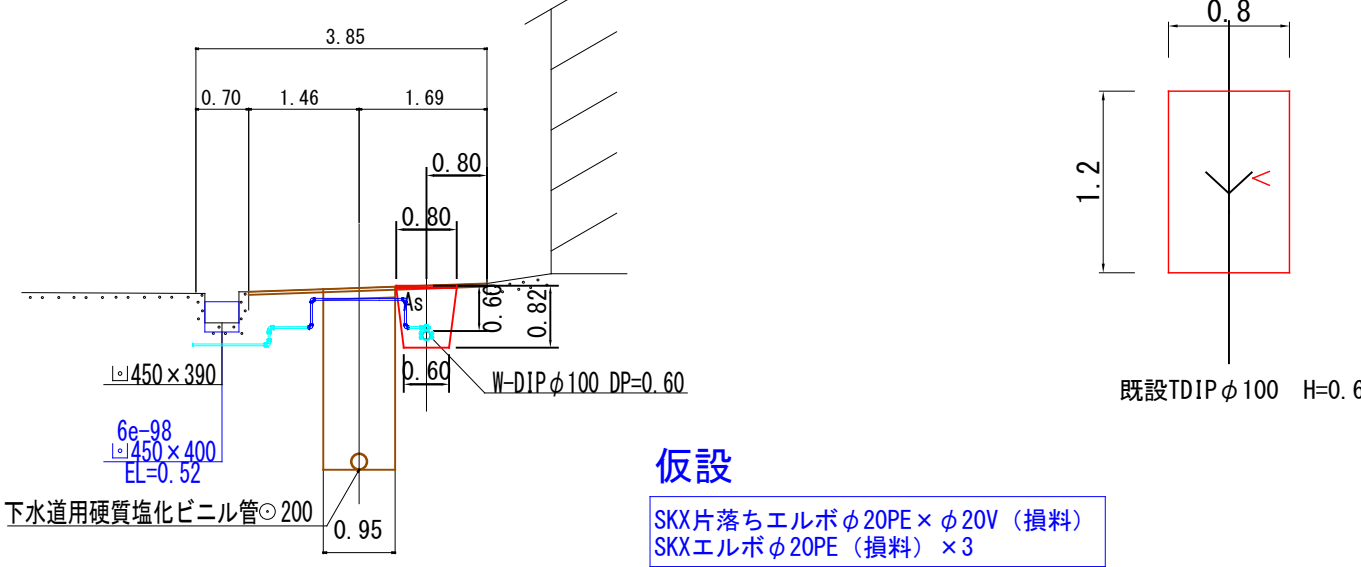
標準掘削断面図
