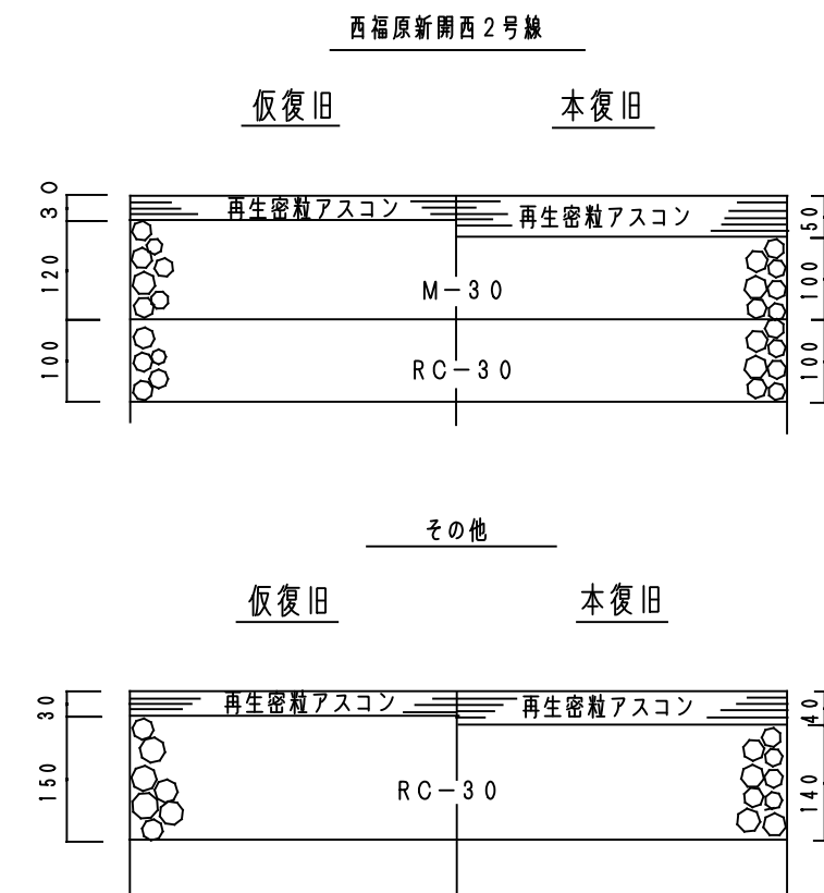
舗装復旧構成図 S=1:10
