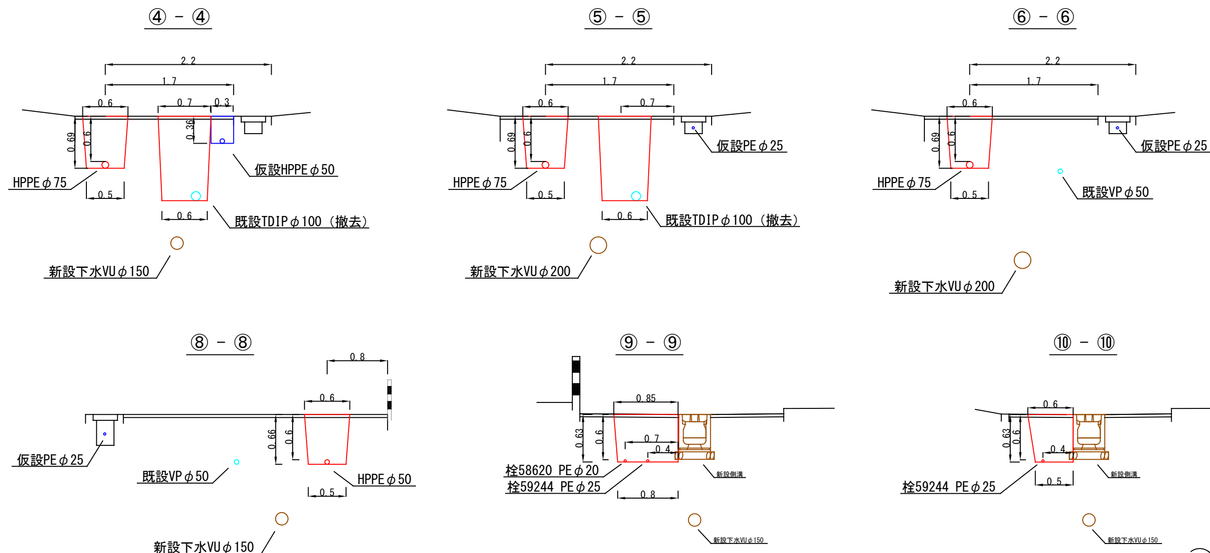
横断面図 S=1:50
