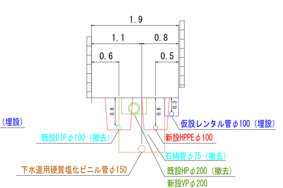
断面図 縮尺1/50
