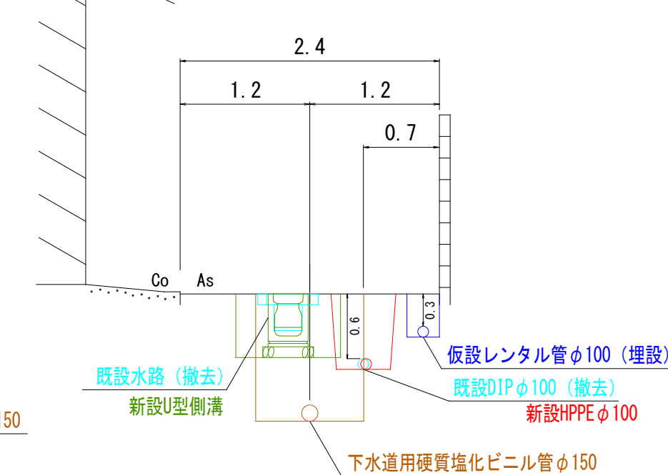
断面図 縮尺1/50
