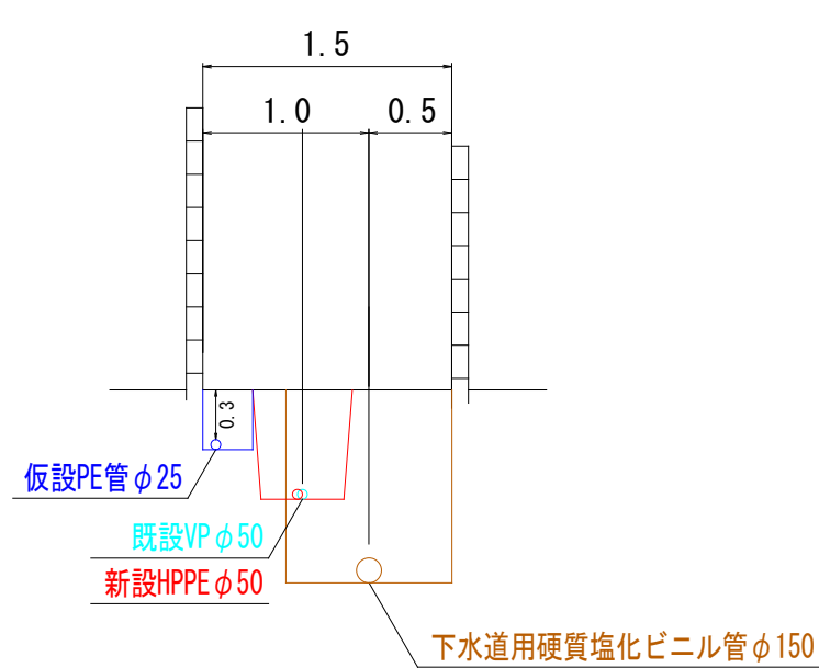
断面図 縮尺1/50
