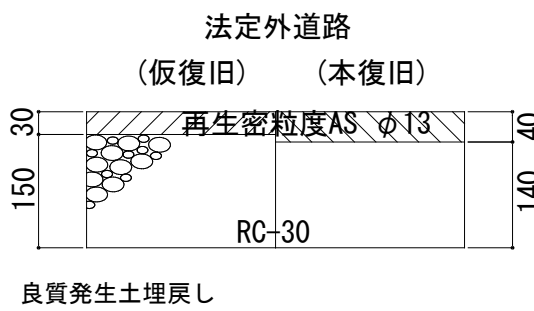
舗装復旧構成図 S=1:10
