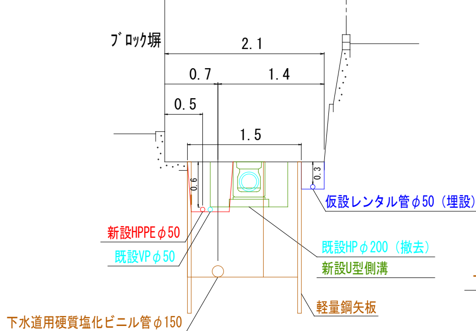
断面図 縮尺1/50
