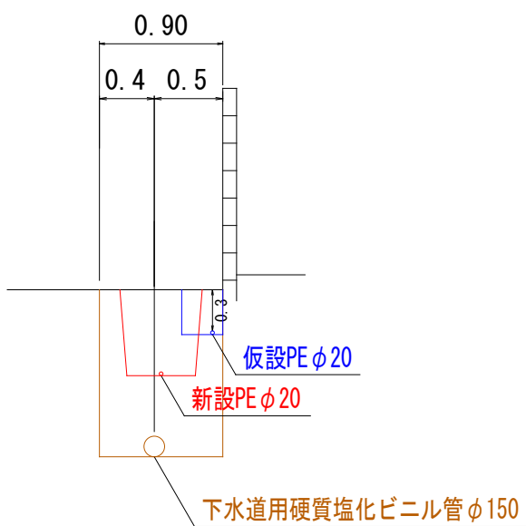
断面図 縮尺1/50
