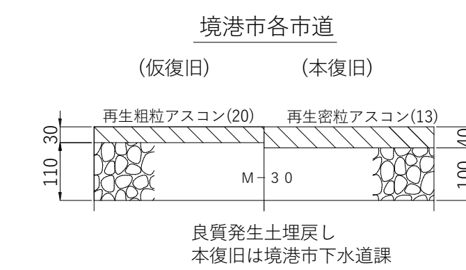
復旧構成図 S=1/10
