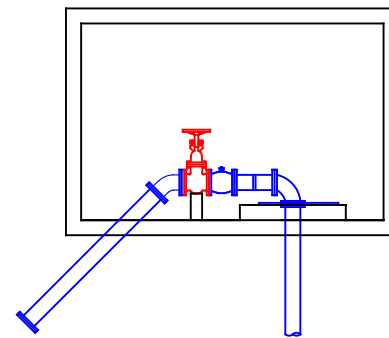
取水井室断面図
