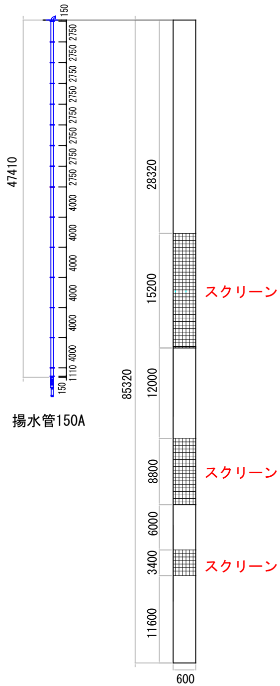
日下水源地取水井詳細図 S=1:500
