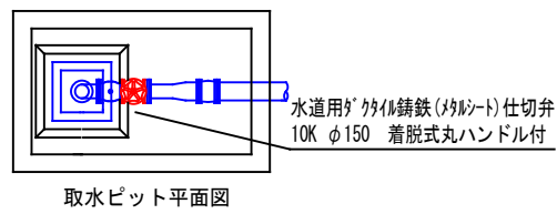
取水ピット平面図
