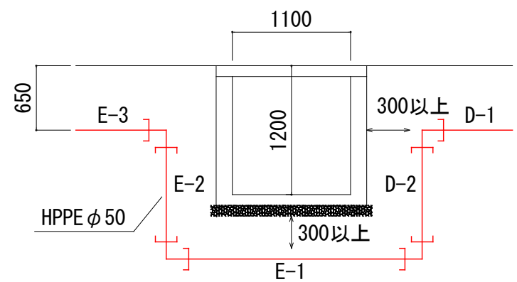
B-B' 伏越し断面図 縮尺1/50
