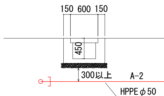
A-A' 伏越し断面図 縮尺1/50
