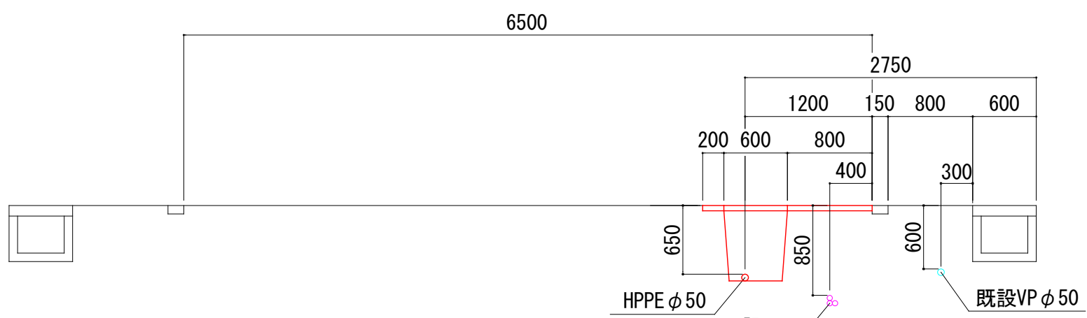
標準断面図 縮尺1/50
