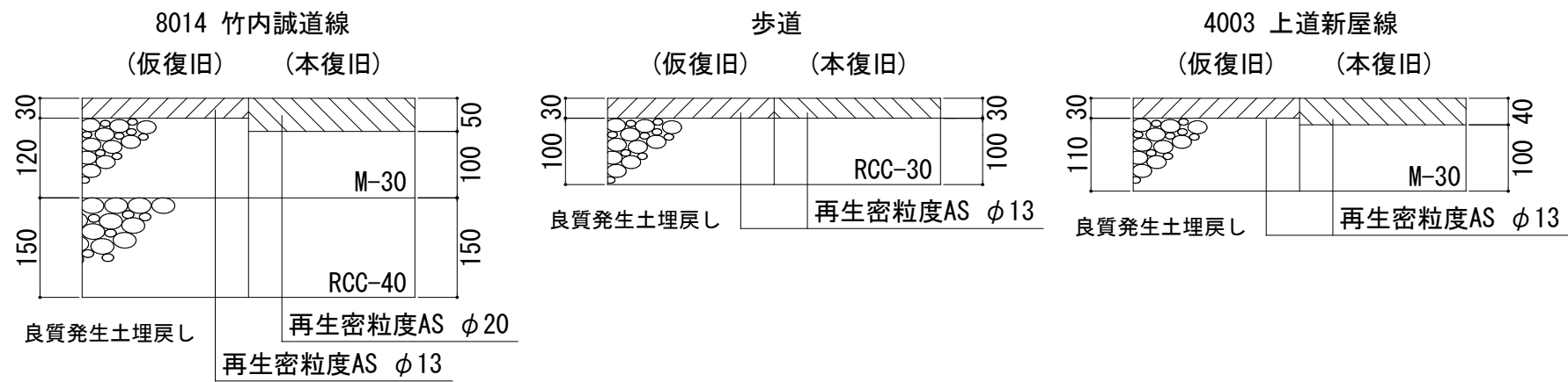
舗装復旧構成図 S=1:10
