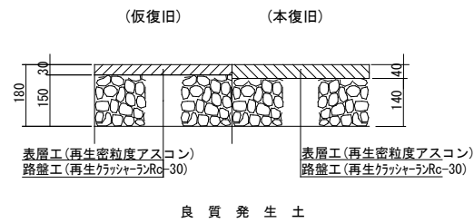
舗装復旧構成図 S=1:10
