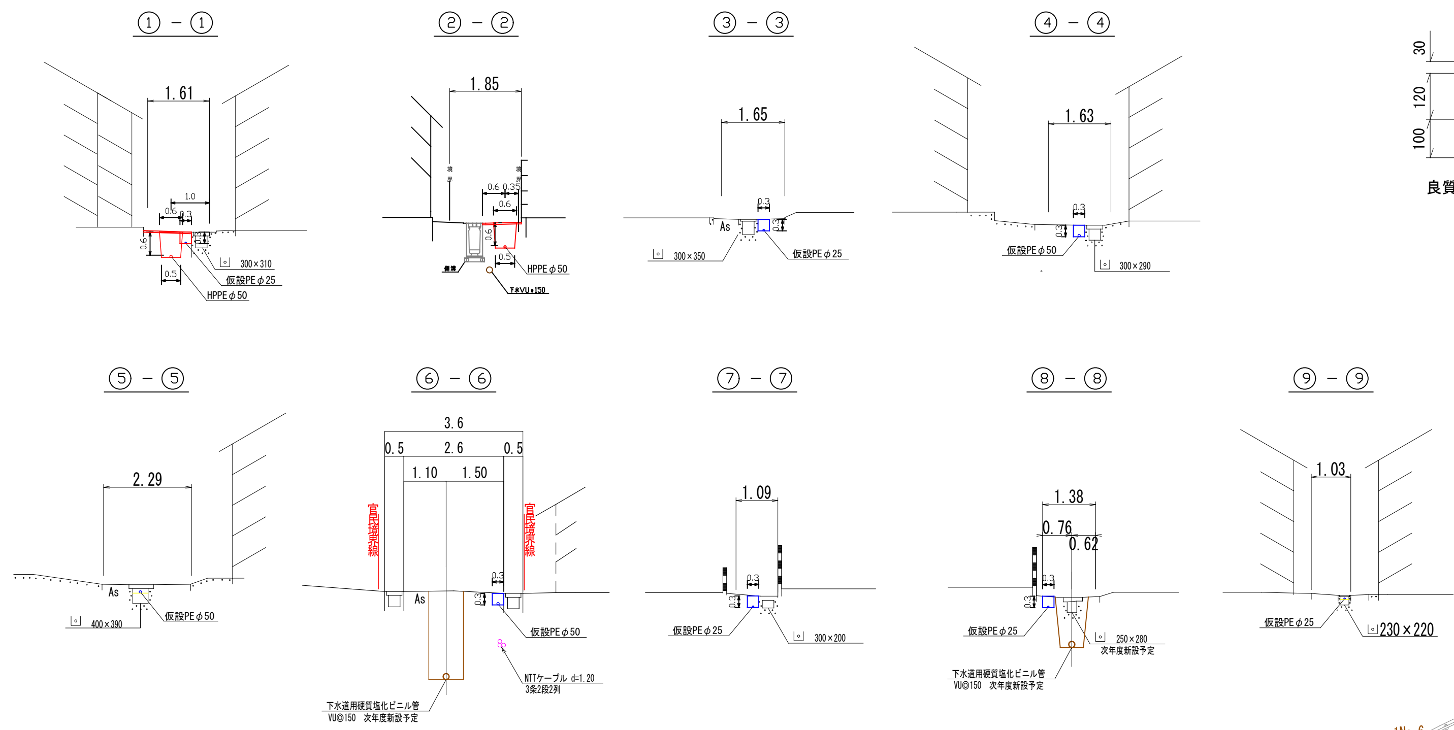
断面図 S=1:100
