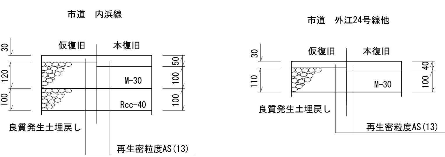
舗装復旧構成図 S=1:10
