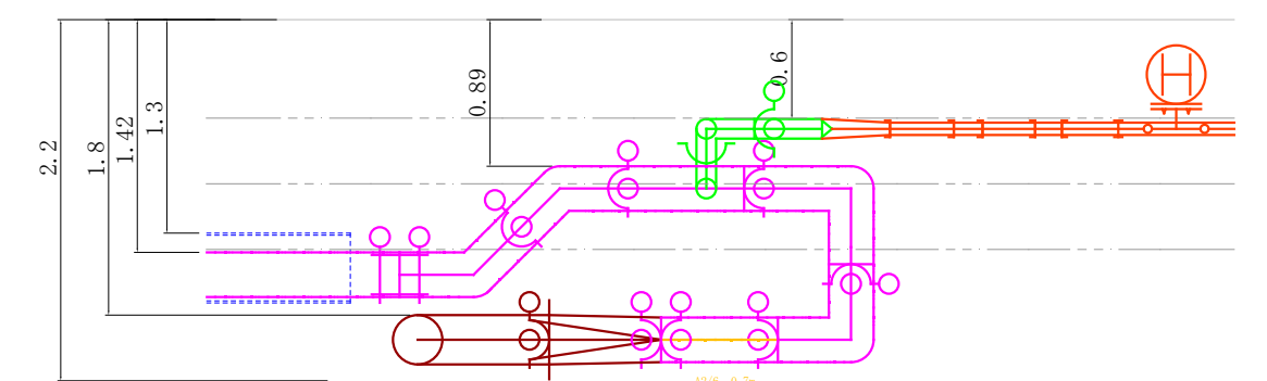
A 断面図 S=1 : 5 0 ( →東側)
