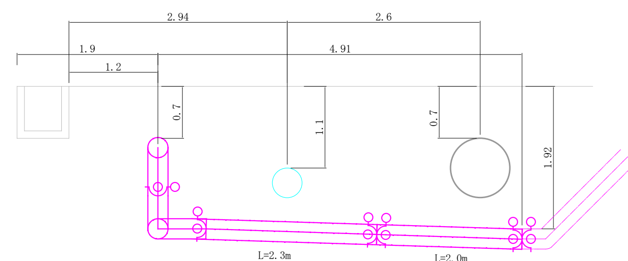
D 断面図 S=1 : 5 0 ( →北側)
