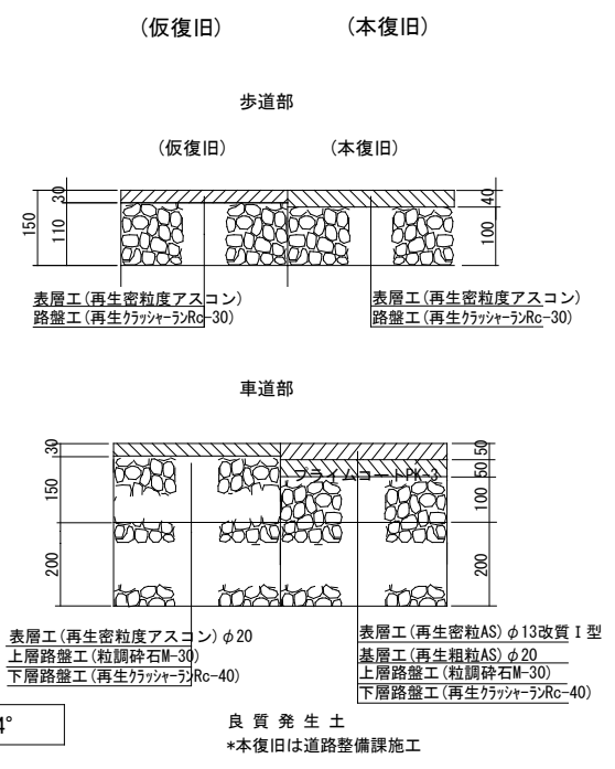
舗装復旧構成図 S=1:10
