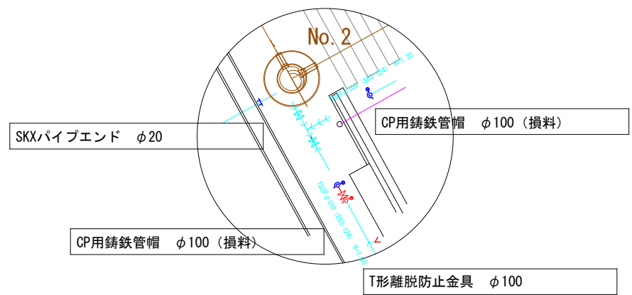
仮設詳細図 S=1:100
