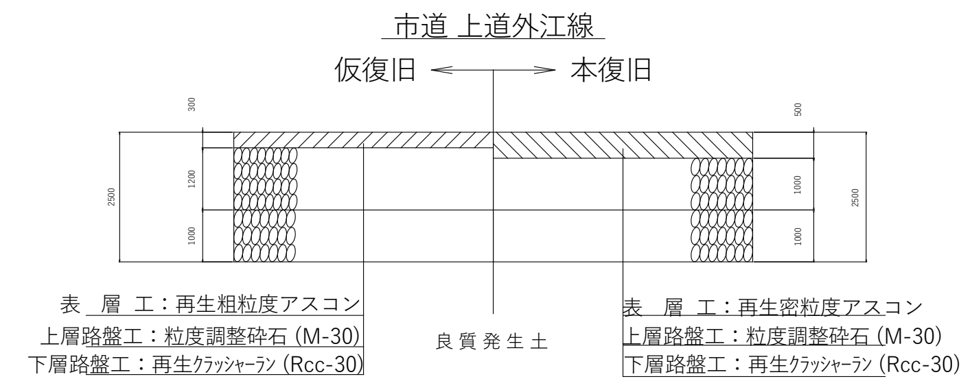
舗装復旧構成図 S=1:10
