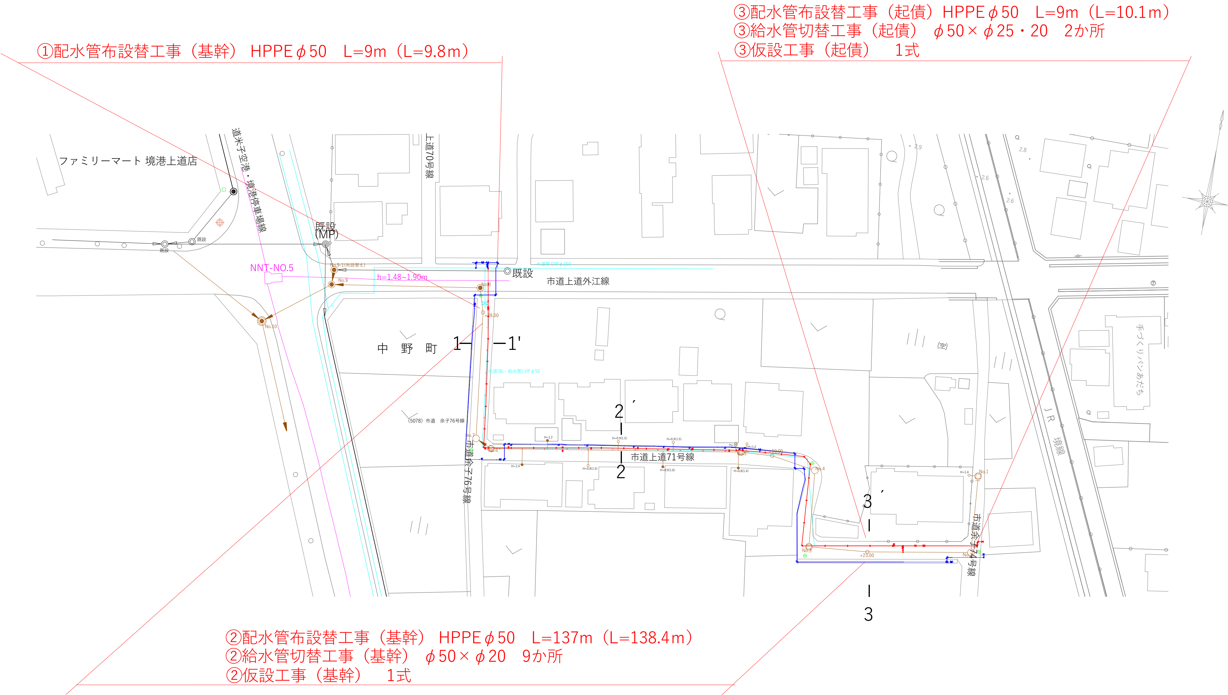
平面図 縮尺 1 : 500
