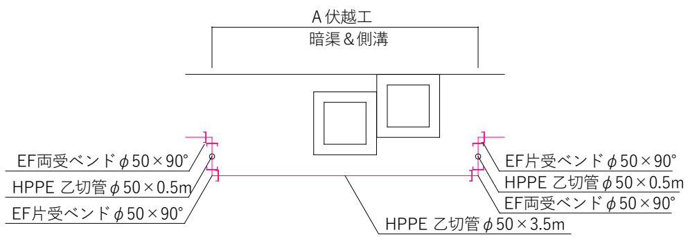
伏越工断面詳細図
