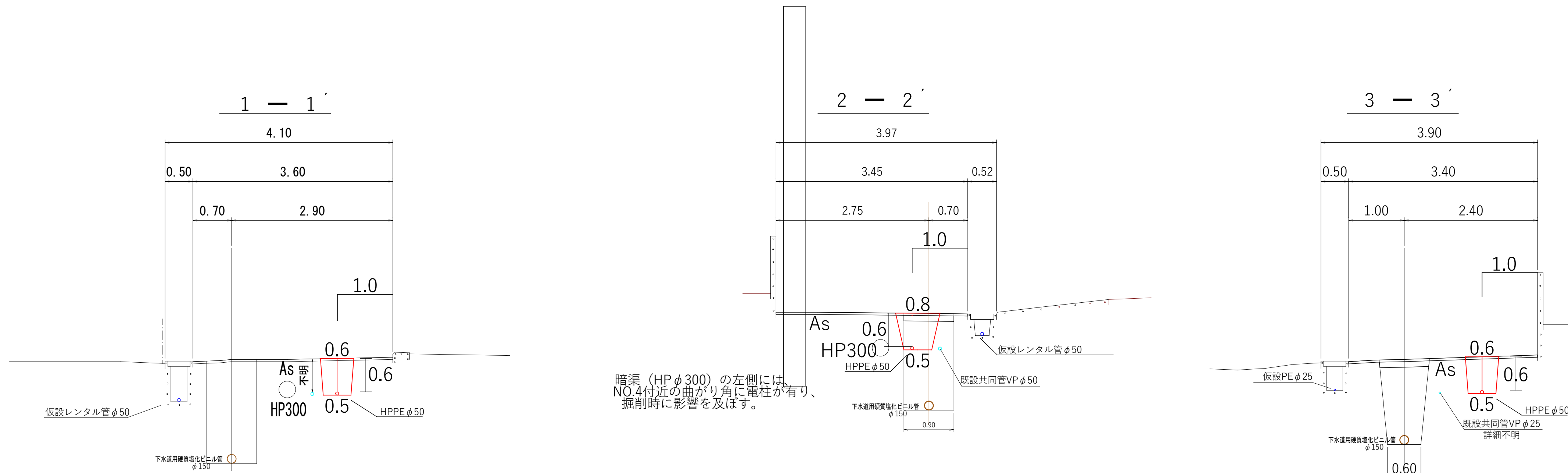
横断面図 縮尺 1:50
