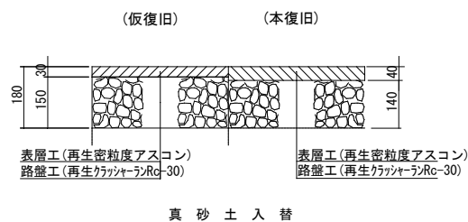
舗装復旧構成図 S=1:20
