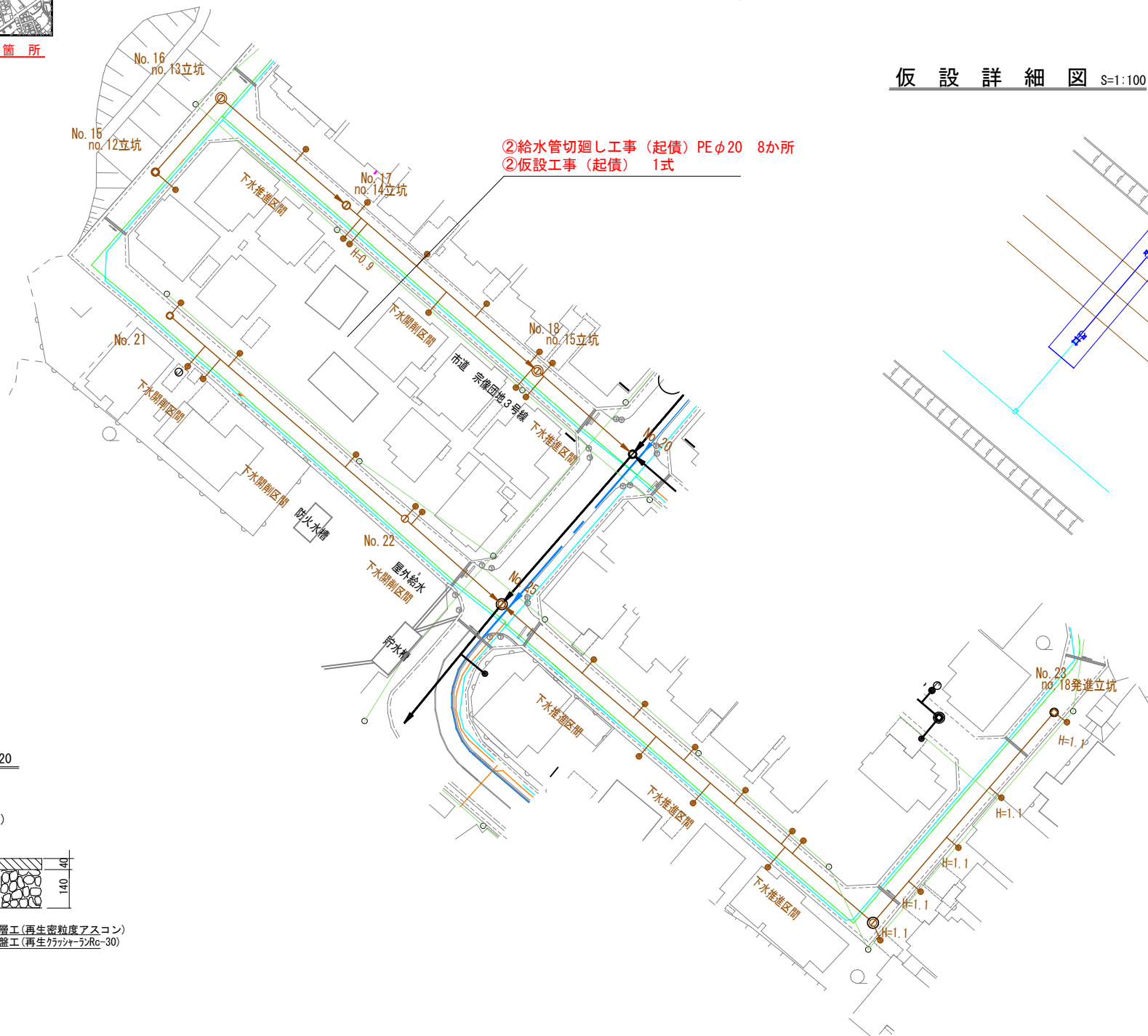
平面図 S=1:1000
