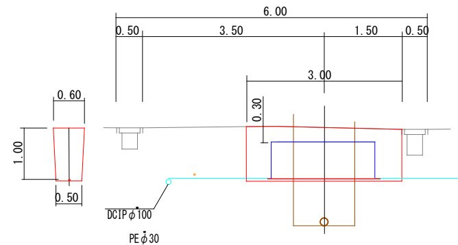
仮設詳細図 S=1:100
