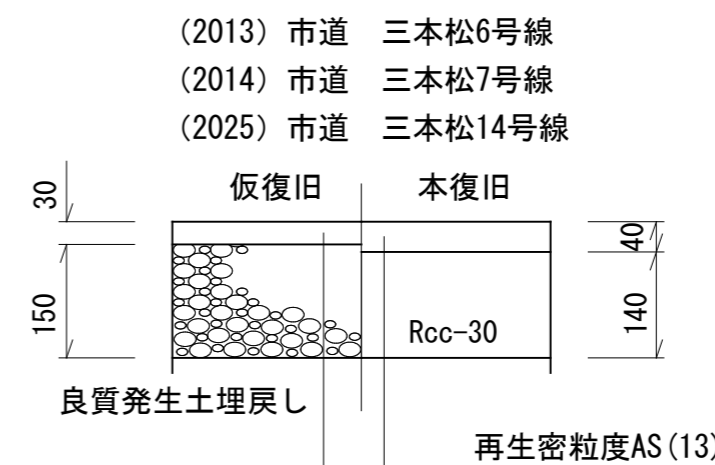
舗装復旧構成図 S=1:10
