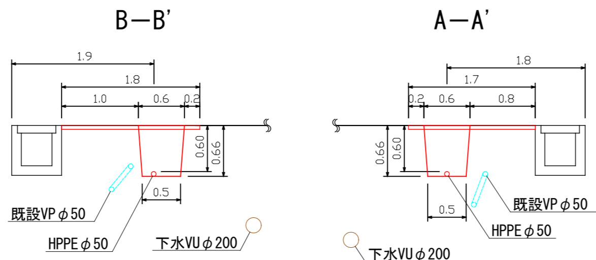
断面図 S=1:50
