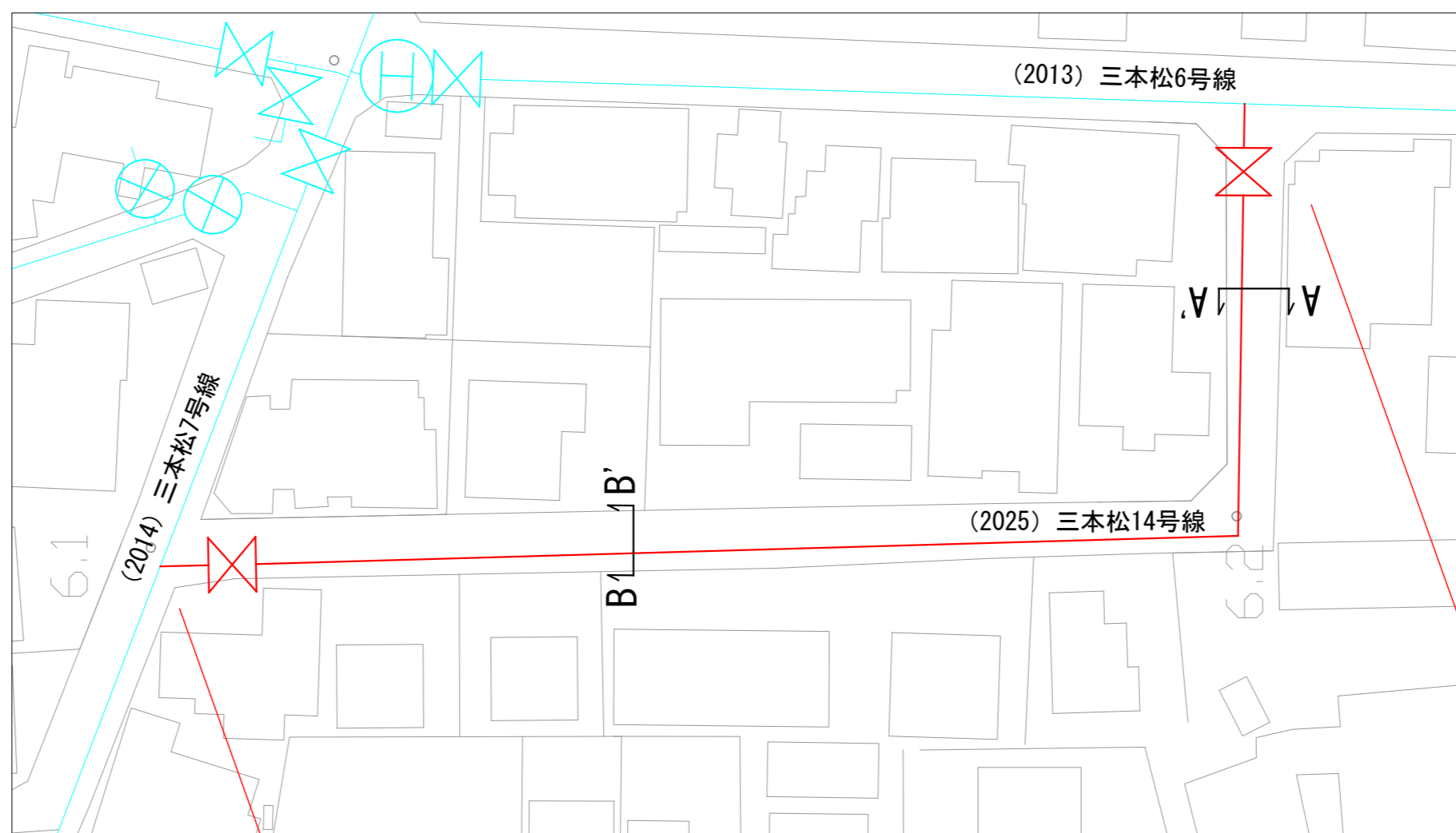
平面図 S=1:500
