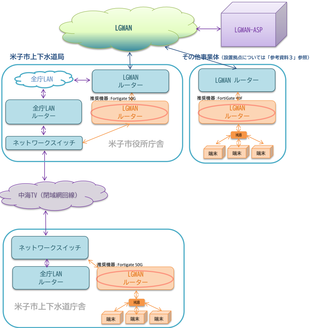
【LGWANを使用する場合の構成イメージ図】
