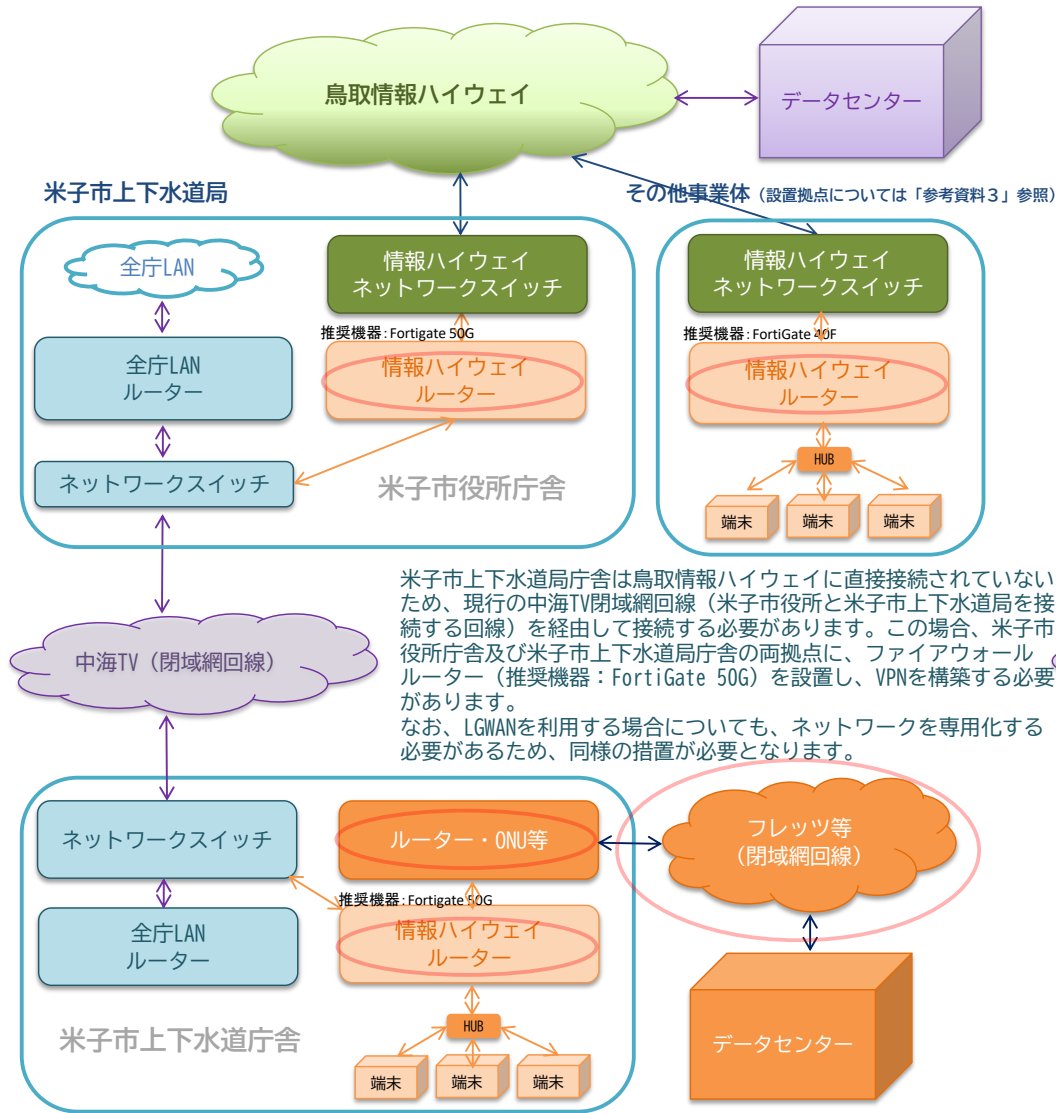
【鳥取情報ハイウェイを介して外部接続する場合の構成イメージ図】
