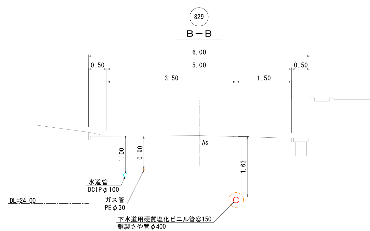
横断面図 縮尺 1:50
