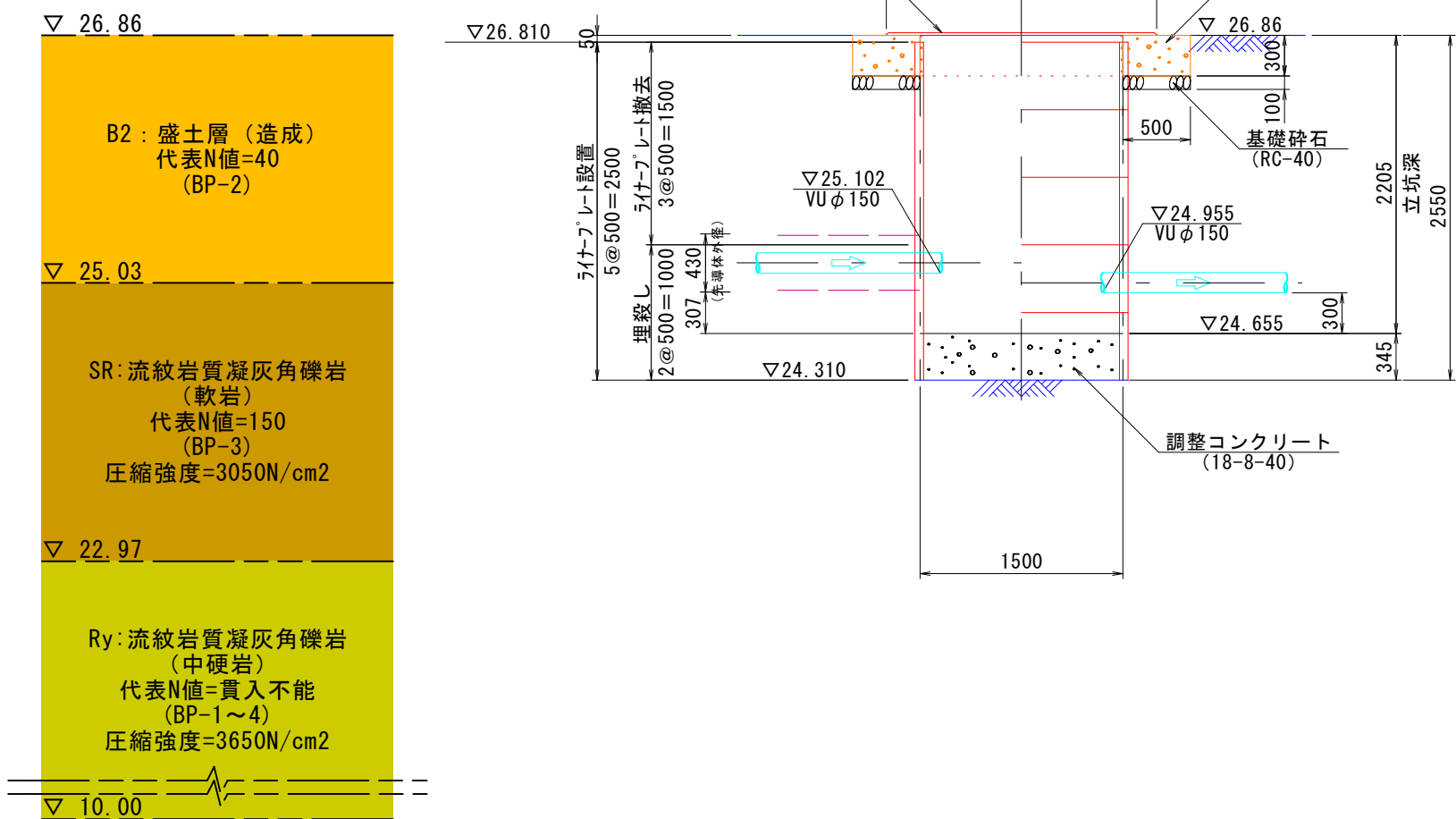
推定土質柱状図
