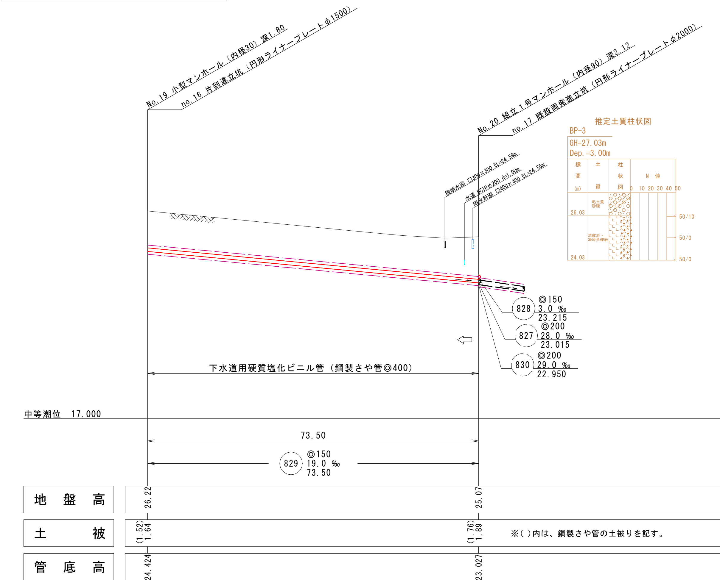
縦断面図 縦縮尺 1:100 横縮尺 1:500
