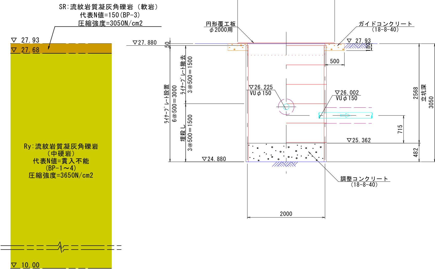
推定土質柱状図
