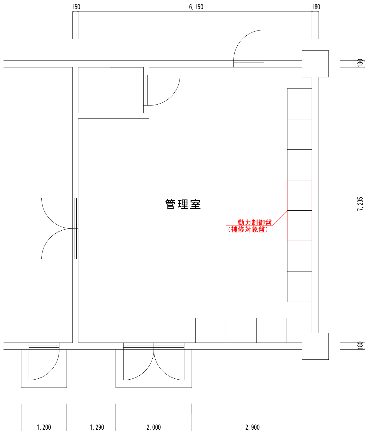
平面図 S:1/60
