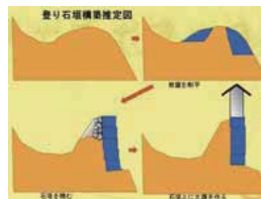
登り石垣の構築推定図
