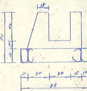
側溝断面图 N=1/30
