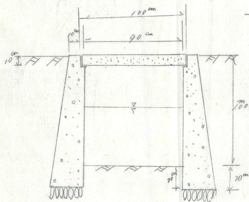
橋断面図
