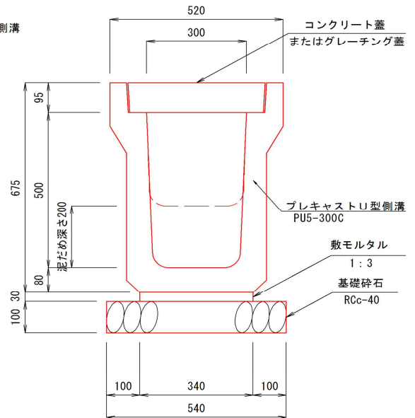
断面図 S=1:10
