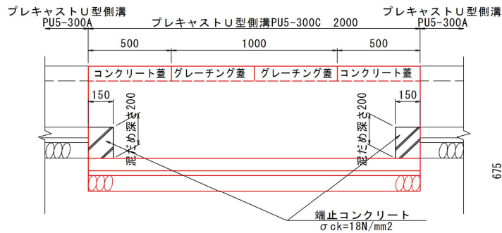
側面図 S=1:20
