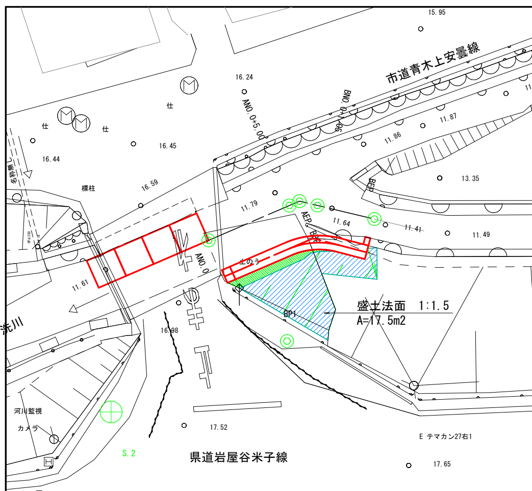
平面图 S=1:200
