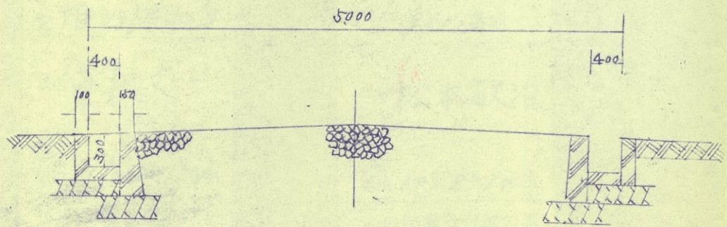
道路標準断面図 S: 1/50
