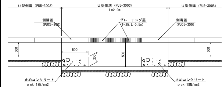
U型側溝(PU5-300C)設置標準図
