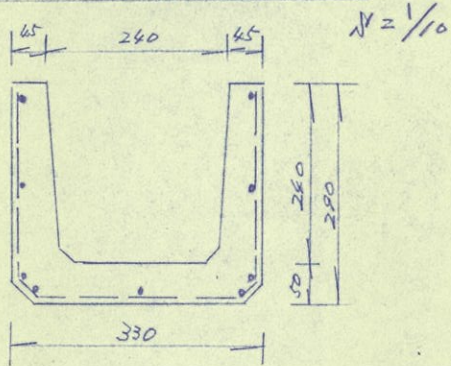
鉄筋コンクリートU型管詳細図 N=1/10
