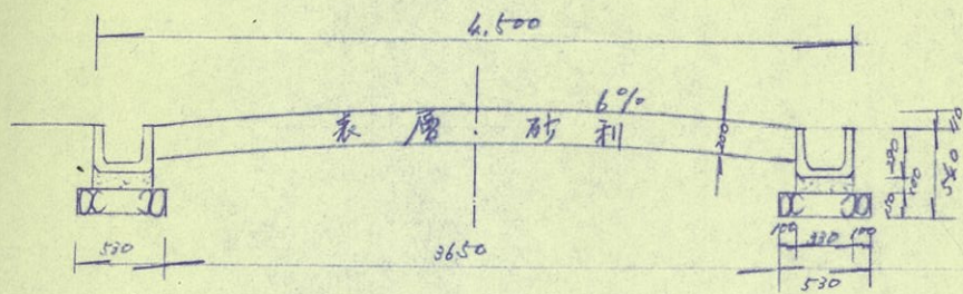
道路標準断面図 N=1/50
