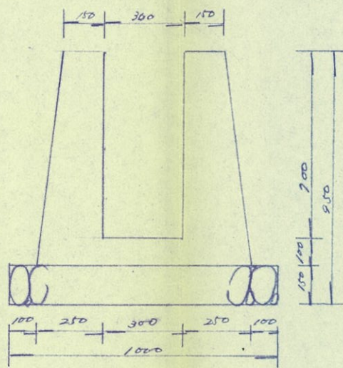
水路標準断面図 N=1/20
