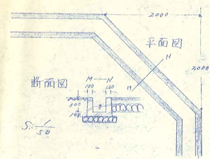
隅切詳細図
