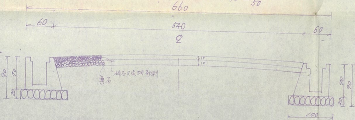
B-B' 標準横断面图
