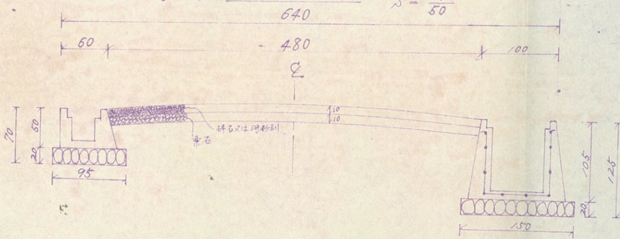
G-G' O-O' 標準横断面图
