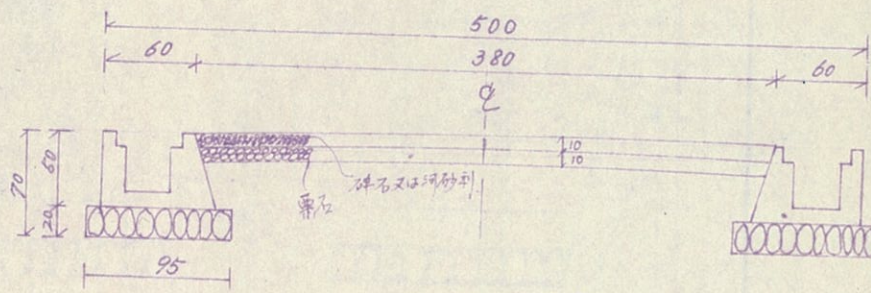
C-C' 標準横断面图
