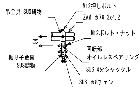
ブランコ回転部詳細図 1 : 2 0
