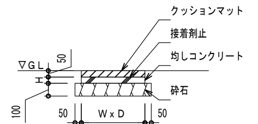
C 詳細図
