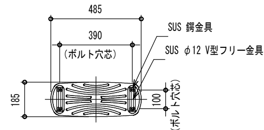
ブランコ踏板詳細図
