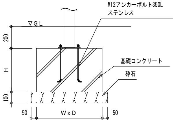
A 詳細図
