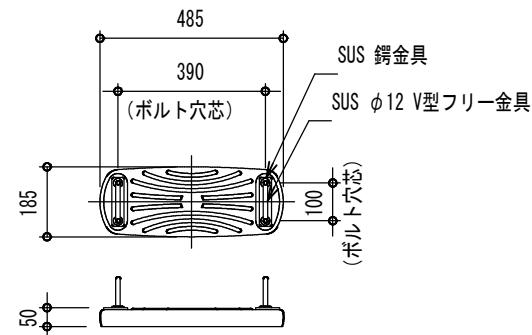
ブランコ踏板詳細図 1 : 2 0
