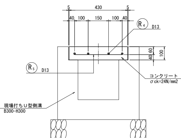
A-A断面図
