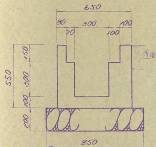
側溝工 S=1:20
