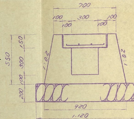
横断暗渠工 S=1:20
