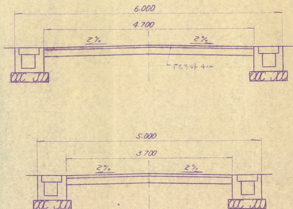
道路断面図 S=1:50
