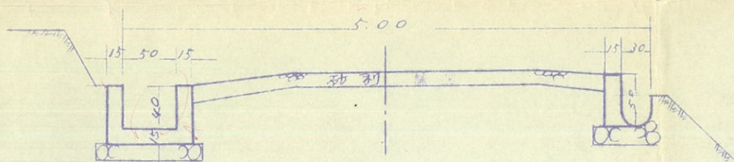
道路定規図 道路 №5 B-B'
