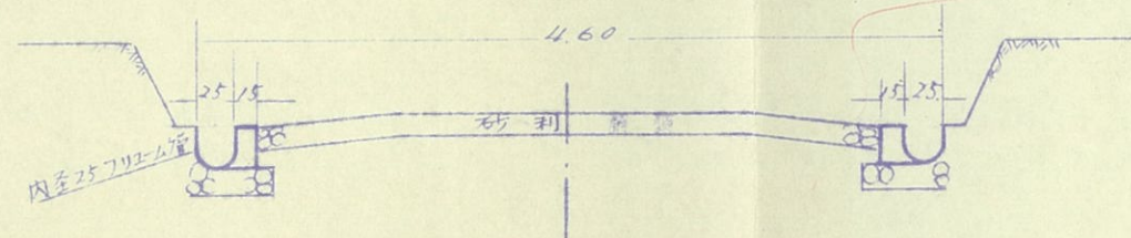
道路定規図 道路 №7~№21
