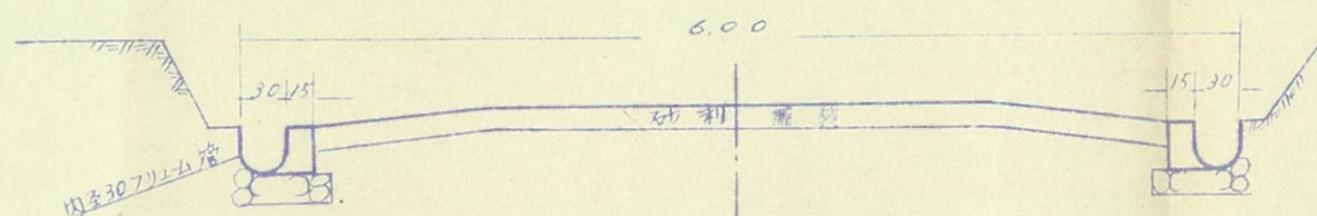
道路定規図 道路 №4
