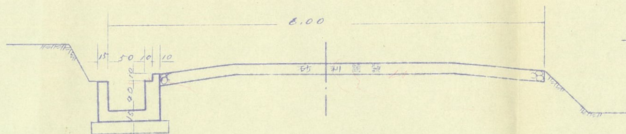
道路定規図 道路 №3 №2
