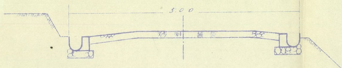
道路定規図 道路 №5 A-A'
