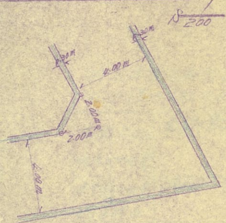
道路指定角切り図
