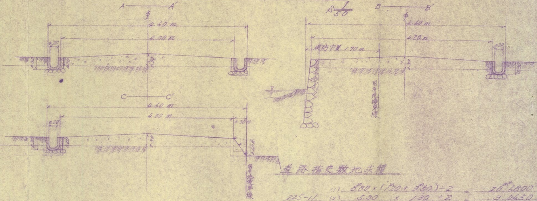
道路標準断面図
