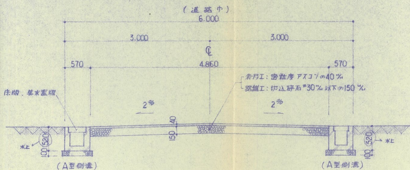
a-a'道路断面図 s = 1/50
