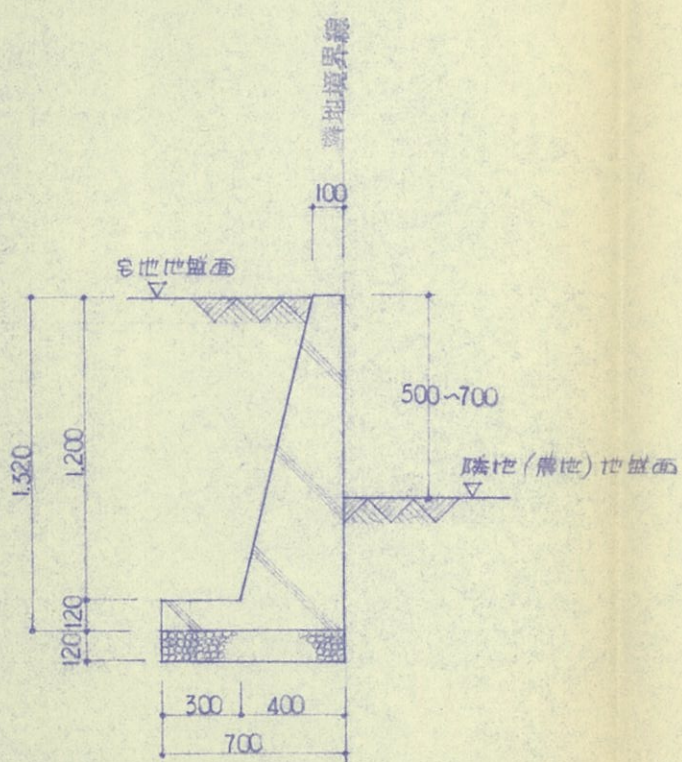
擁壁断面図 s = 1/30
