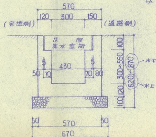
A型側溝断面図 s = 1/20
