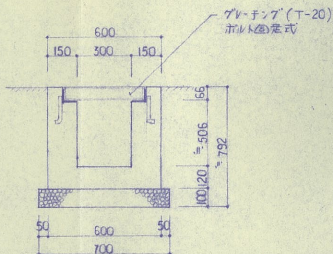
B型側溝 (道路横断面) 断面図 s = 1/20
