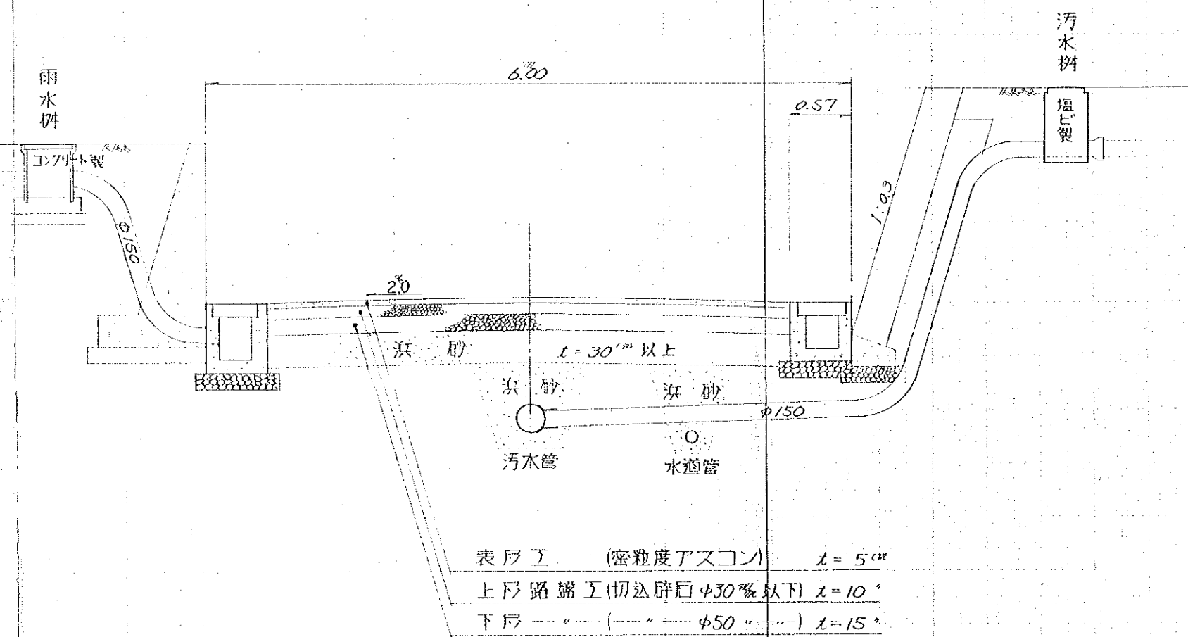
団地間回遊路 標準断面図 縮尺 1:50
