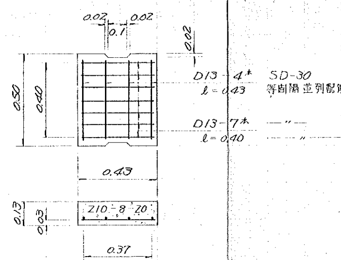
側溝蓋 T20
