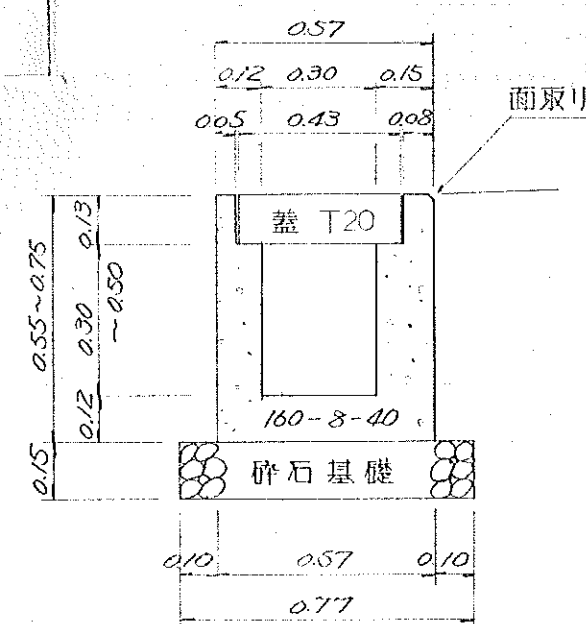
車道用側溝
