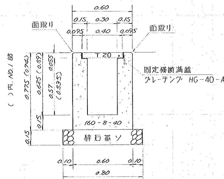
横断側溝
