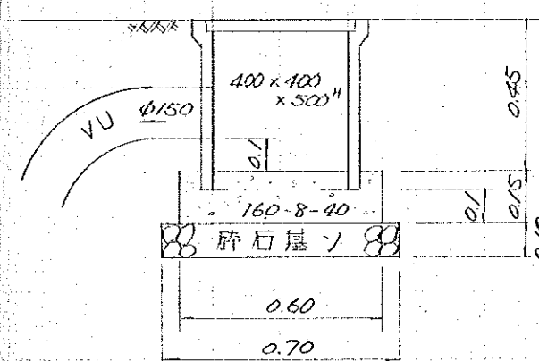
雨水枡
