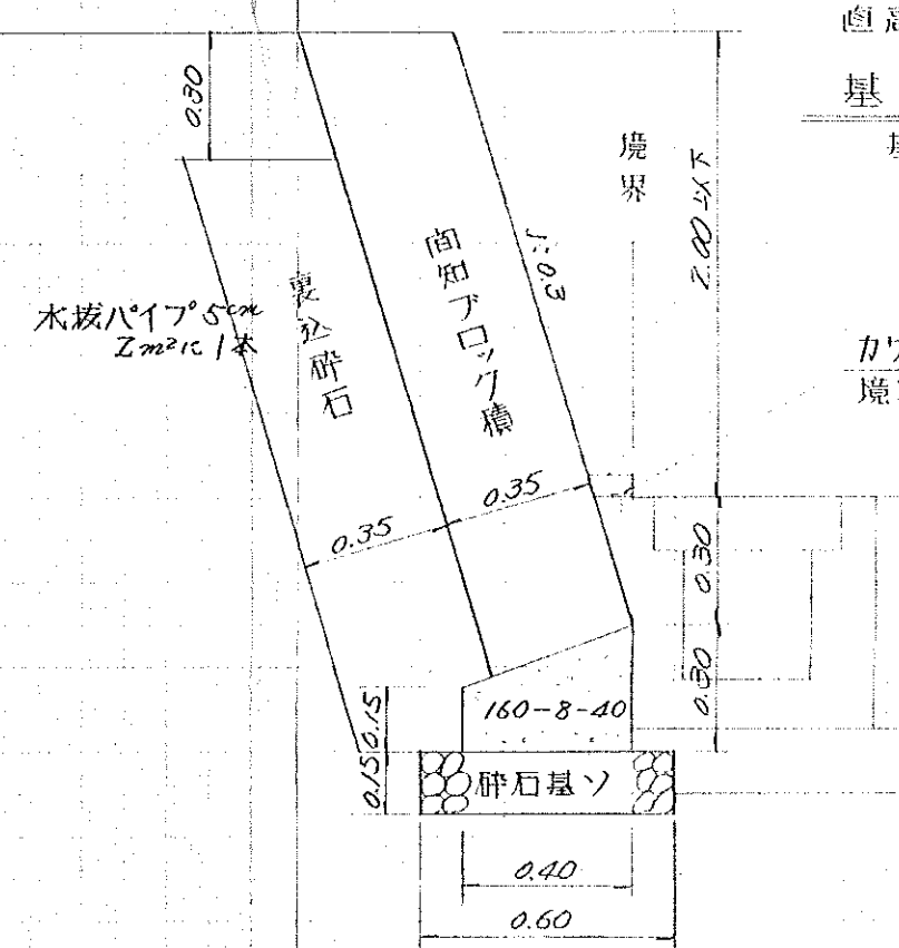
直高 2.0m 以上 基礎Ⅰ型
