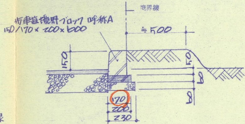
A' 断面図 S = 1/20
