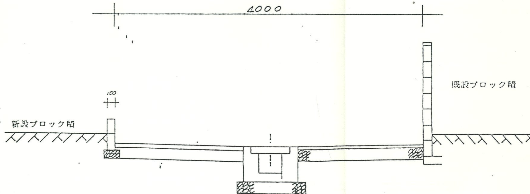
B - B' 断面図
