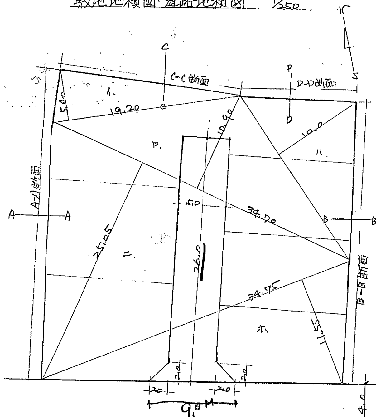
敷地地積図・道路地積図 1/250
