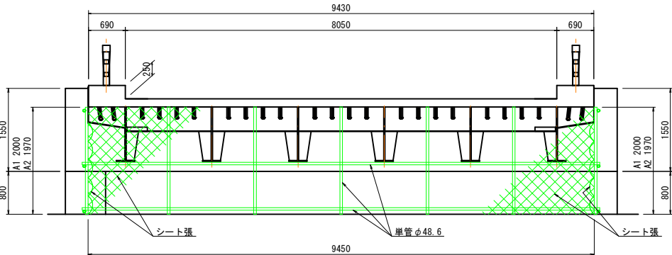
断面図 S=1:50 (防護工)
