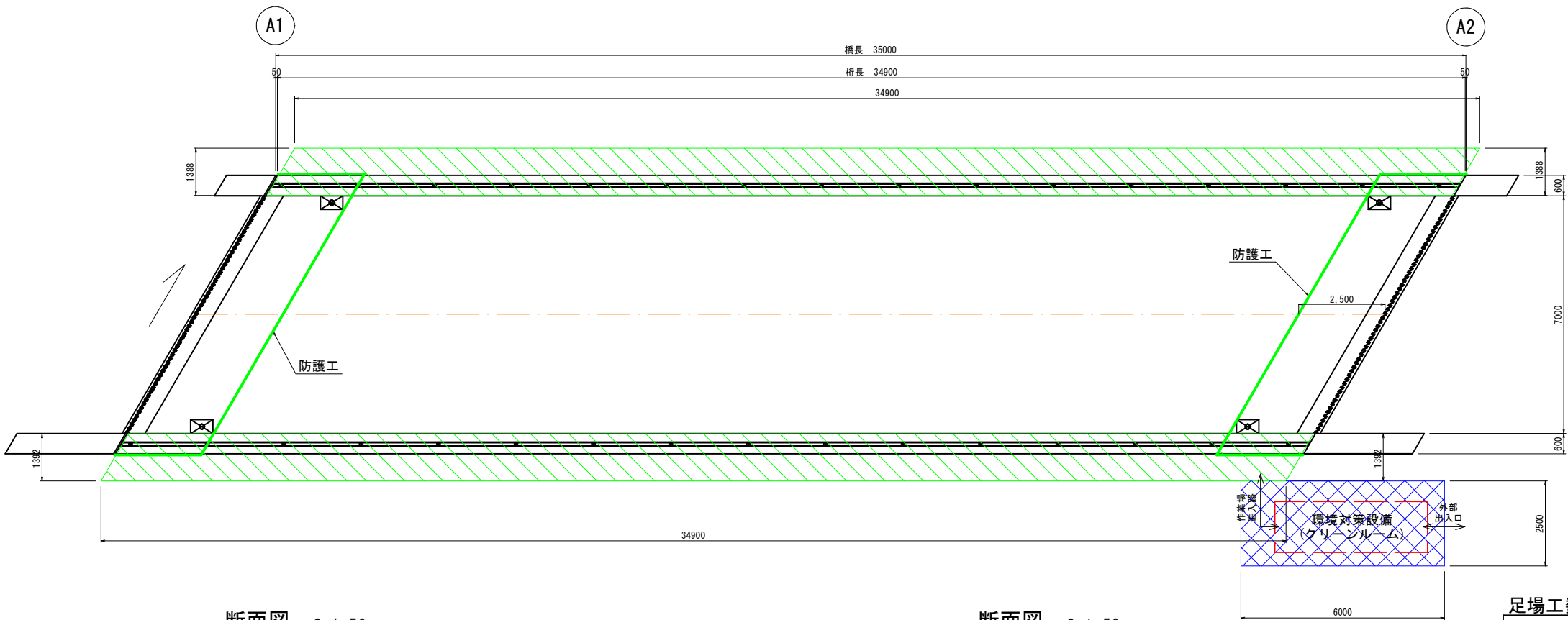
断面図 S=1:50 (防護工)
