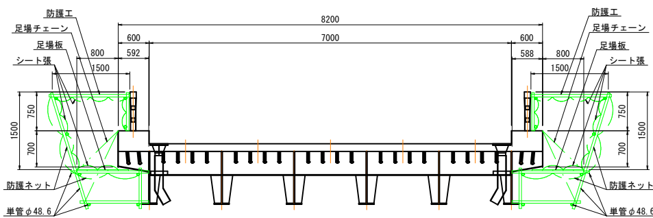
断面図 S=1:50
