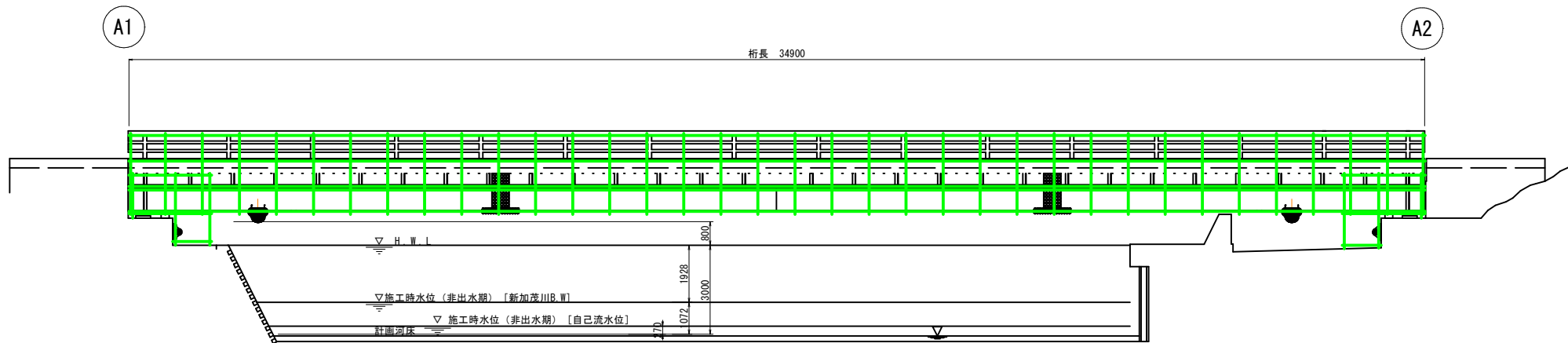
側面図 S=1:80
