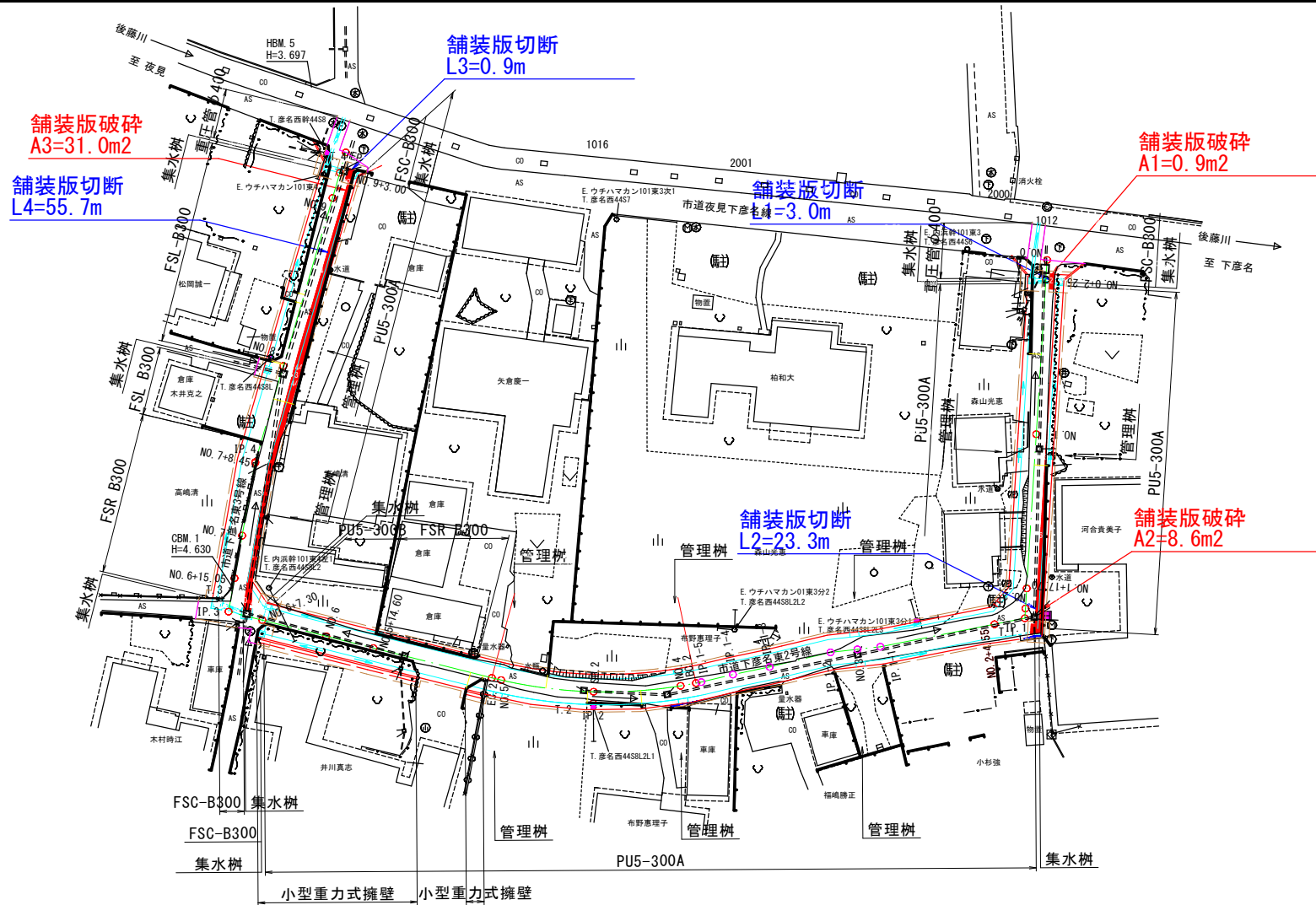
撤去工平面図
