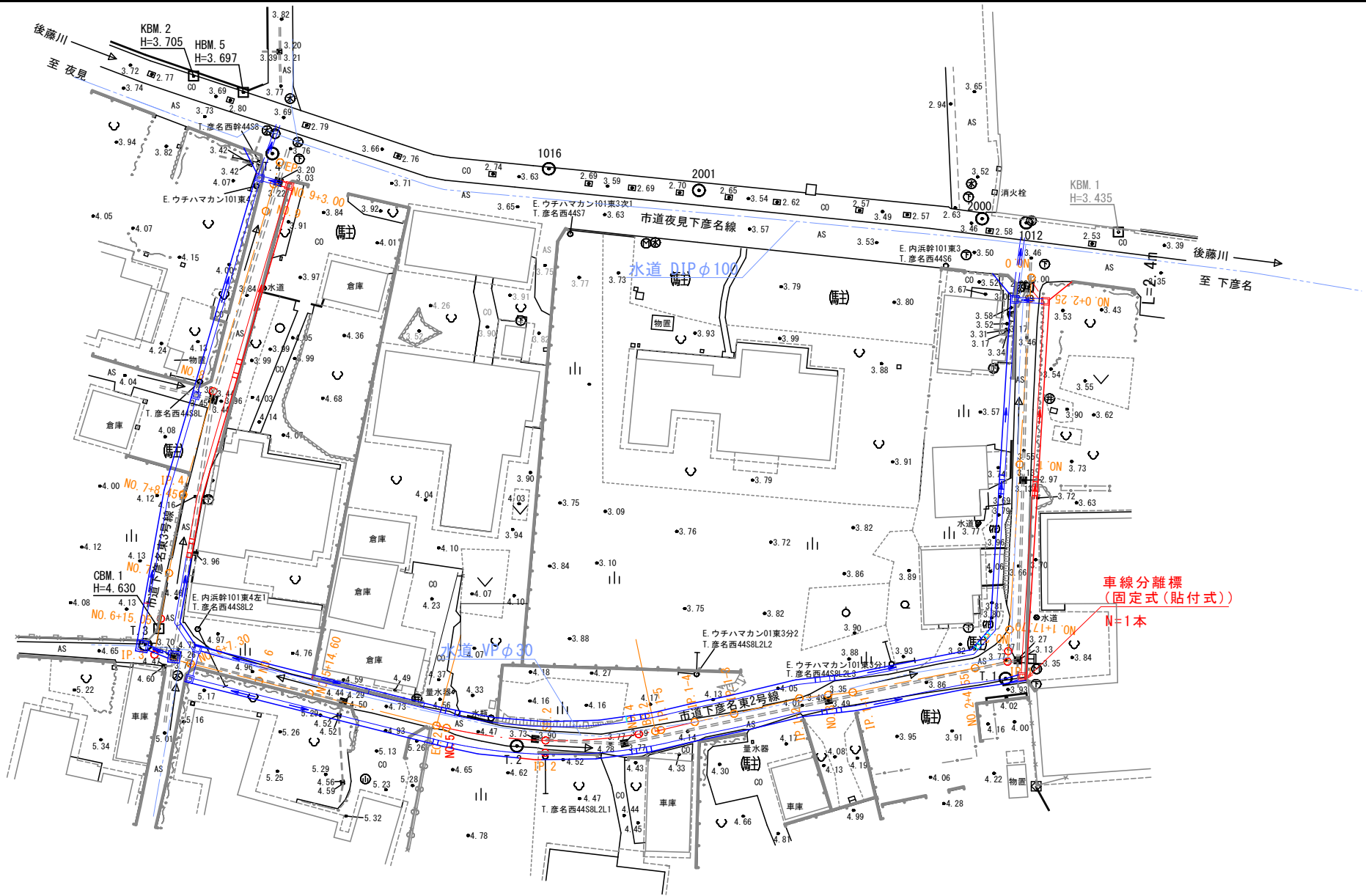
道路附属物工平面図
