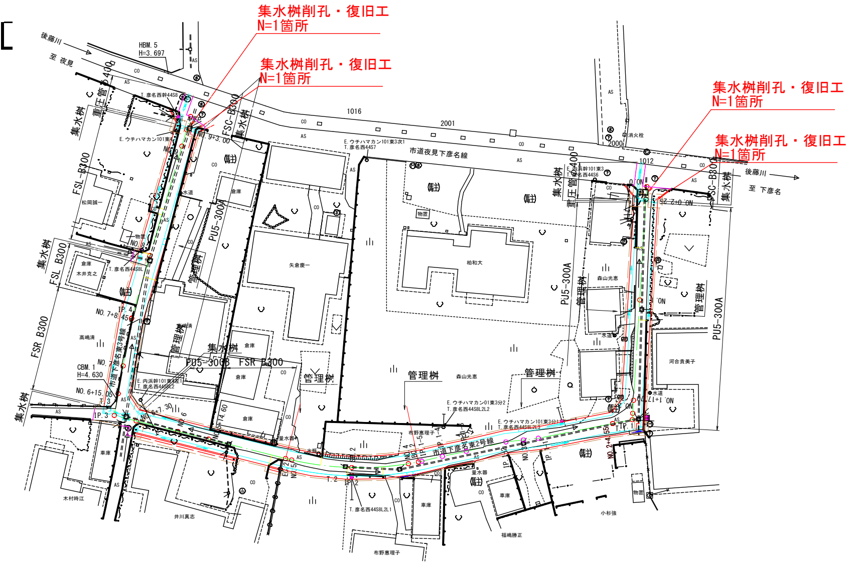
集水樹削孔・復旧工 根拠図
