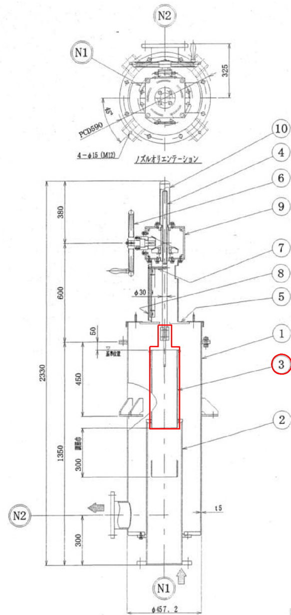
水位調節装置詳細図 NTS
