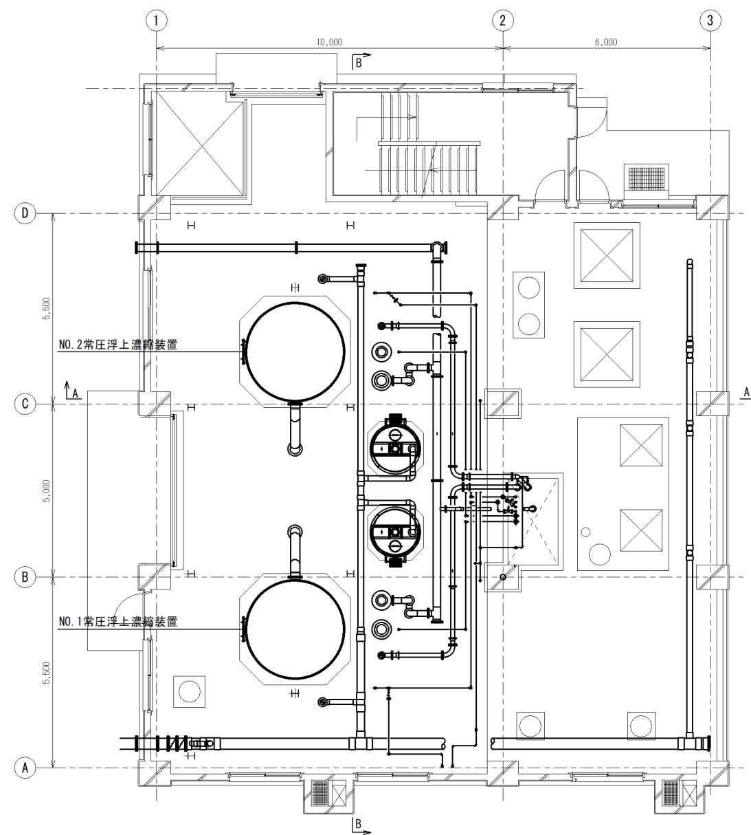
強制濃縮棟1階上部平面図 S:1/150 (A3)
