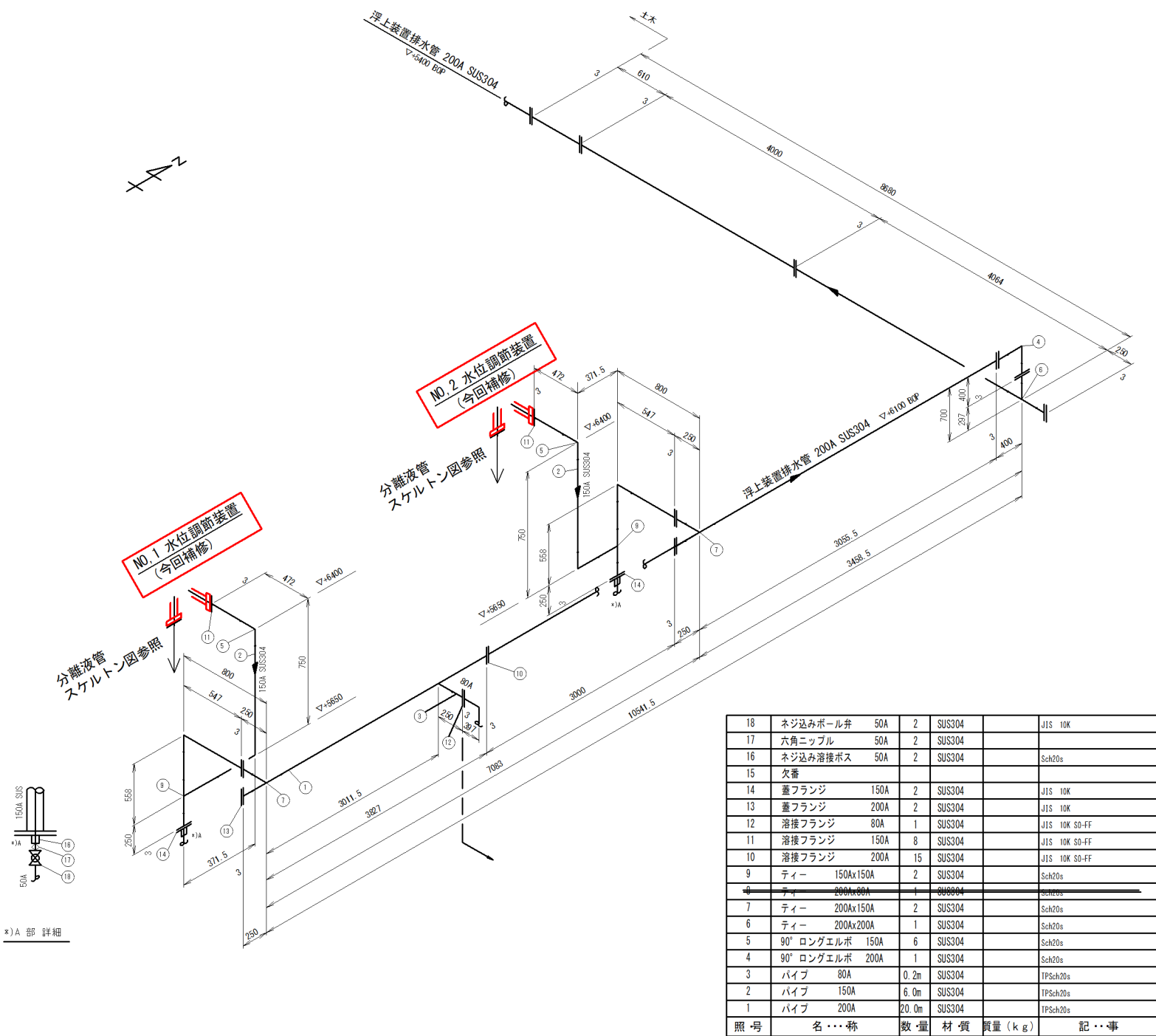
浮上装置排水管スケルトン図 NTS
