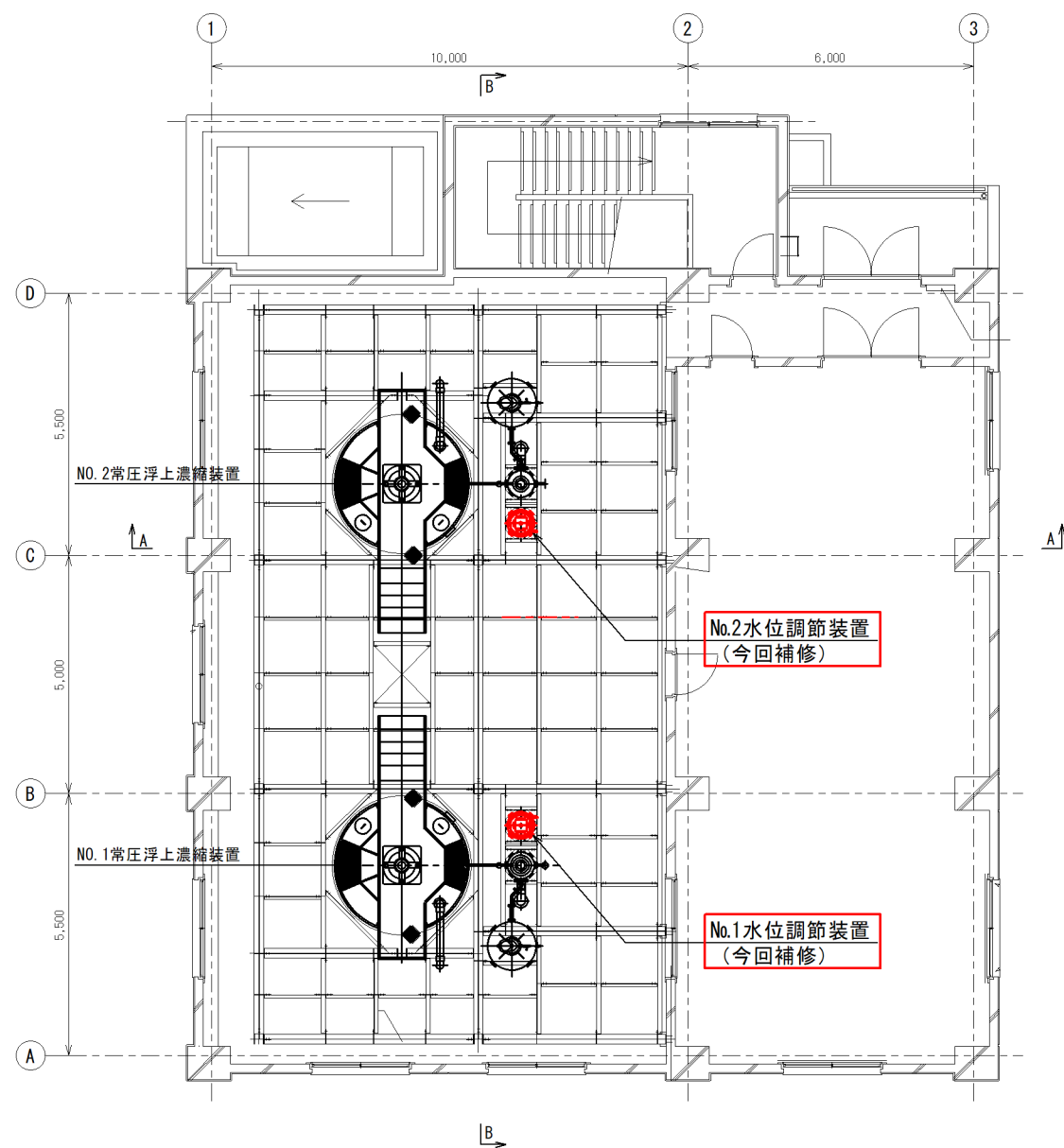
強制濃縮棟2階平面図 S:1/150 (A3)
