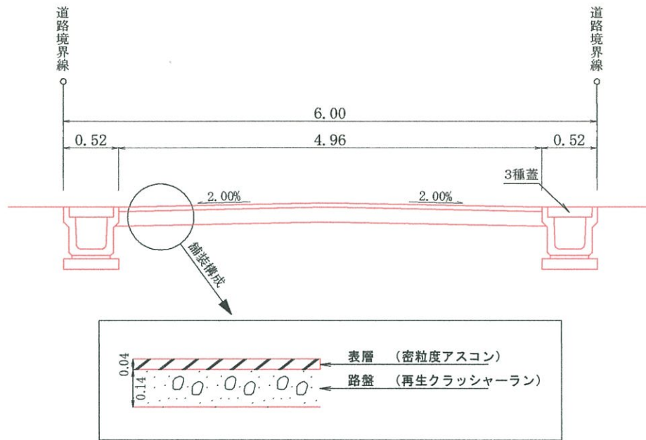
定規図 S=1:50
