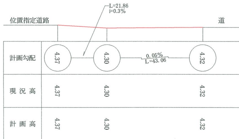
計画縦断面図 S=1:500(縦: 1/50)
