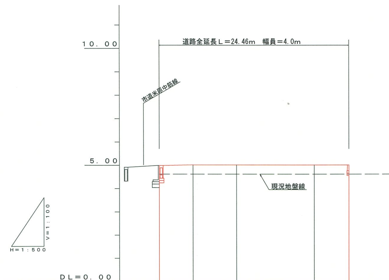
計画道路縦断図
