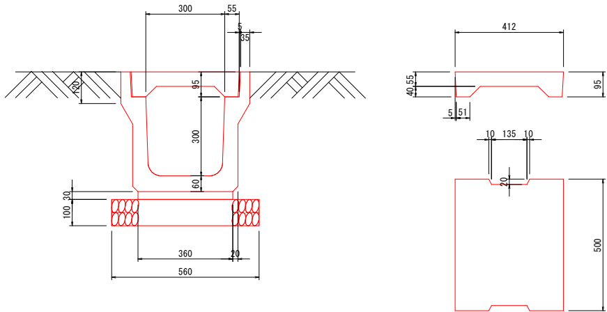
プレキャスト落とし式U型側溝 (1種) PU4 300 10m当り
