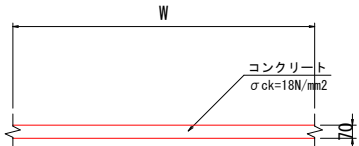
平張コンクリート S=1:20 t=7cm
