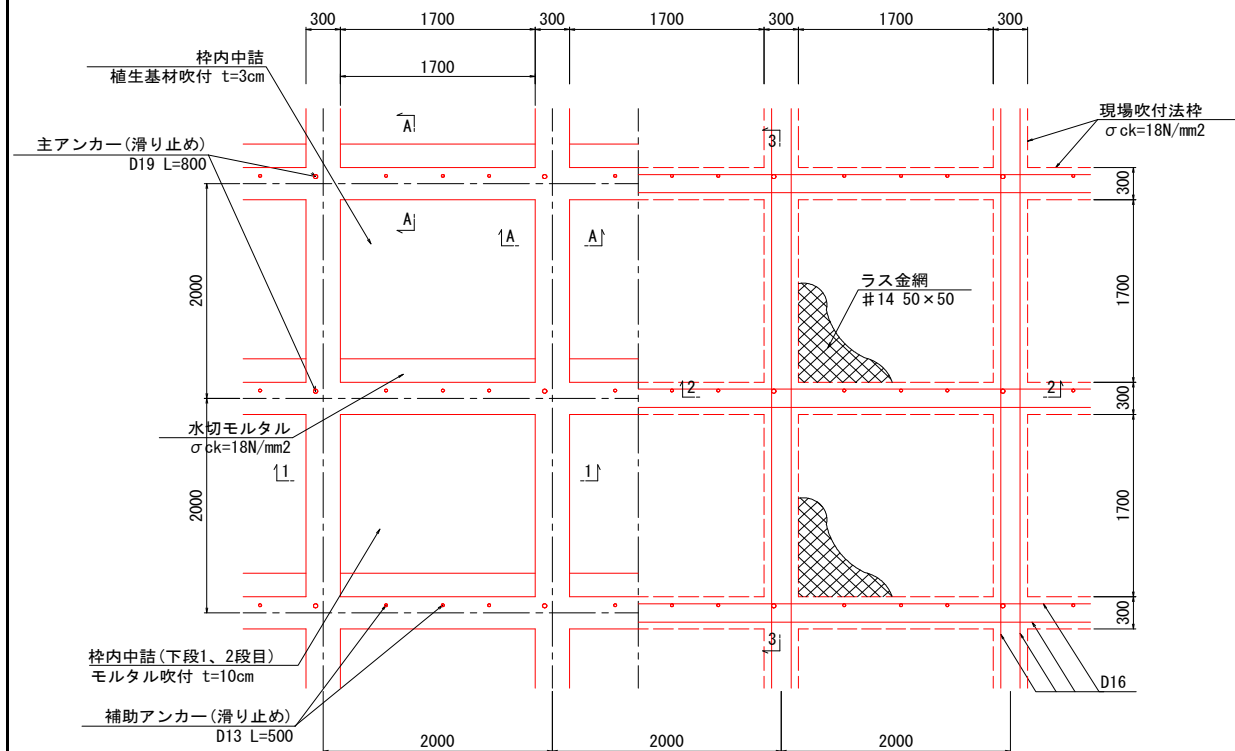
吹付法枠工 (300×300-2000) 数量算出表
