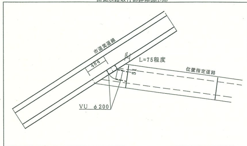
山側水路取付部詳細図(1/50)
