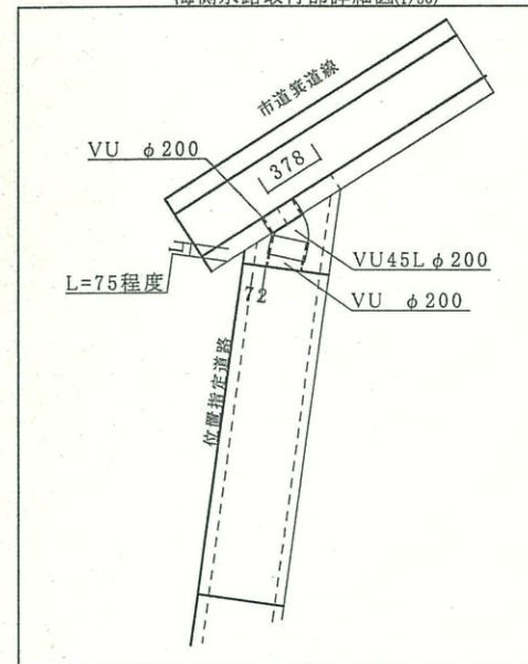
海側水路取付部詳細図(1/50)
