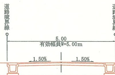
A - A 横断面図 1/100
