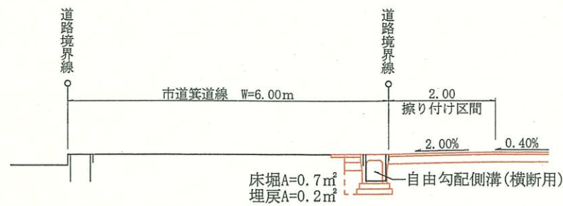
B - B 横断面図 1/100
