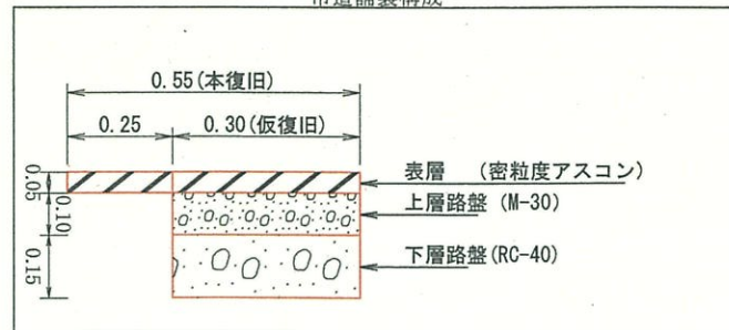
市道舗装構成
