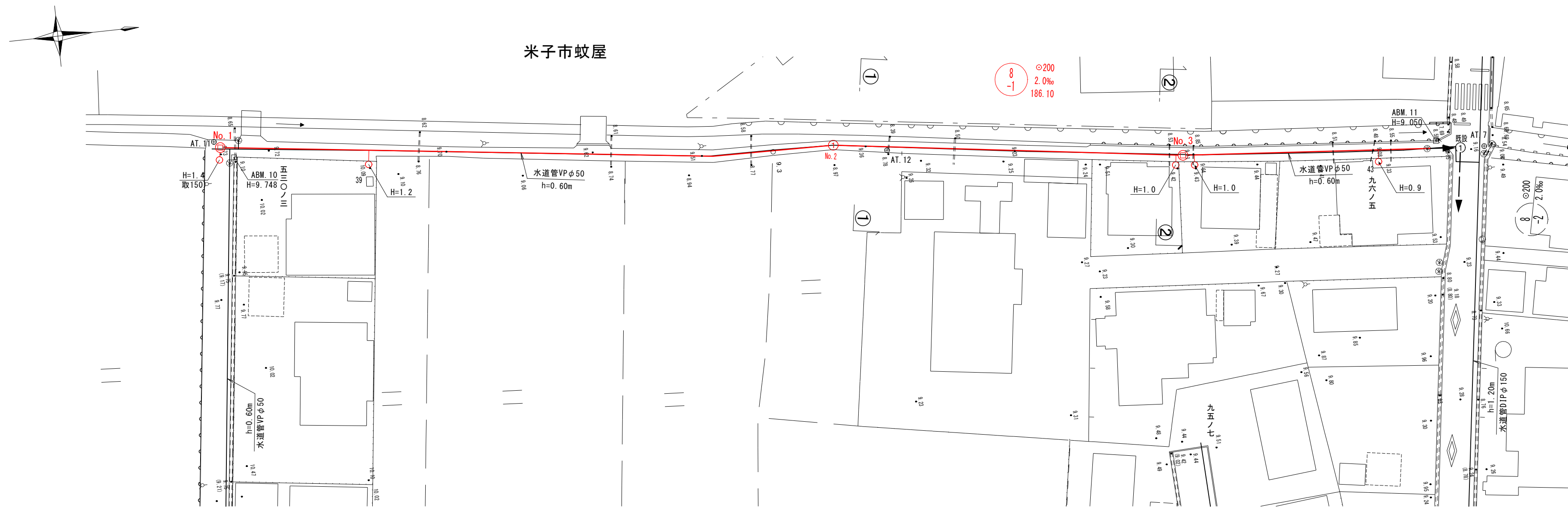
平面図 縮尺 1/500
