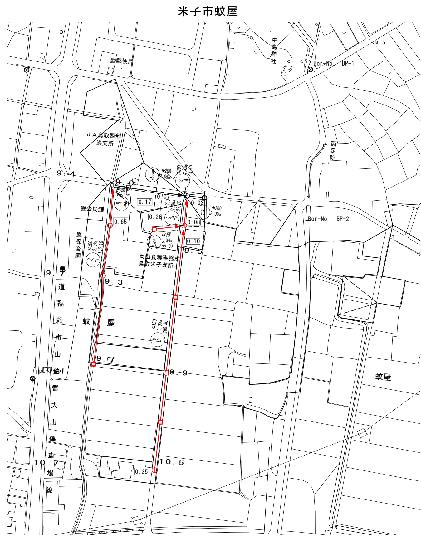
系統図 縮尺 1/2500
