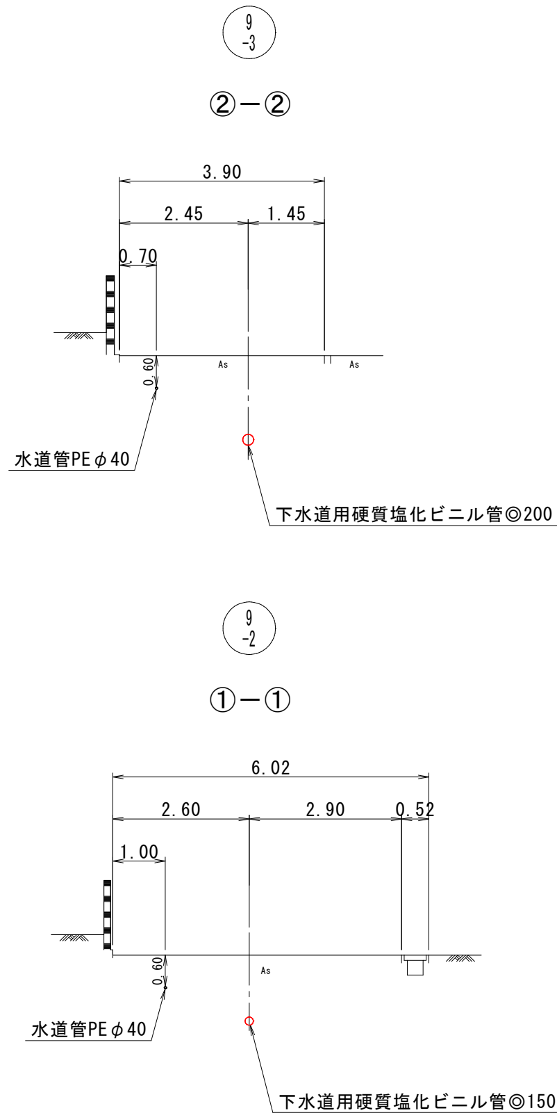
横断面図 縮尺 1/100
