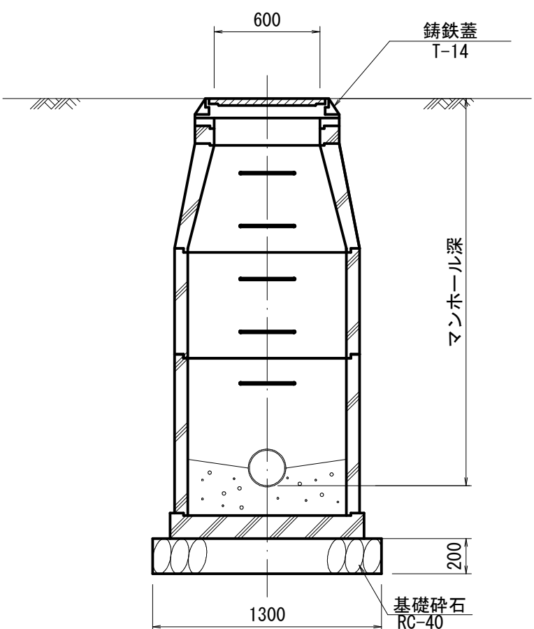
横断面図
