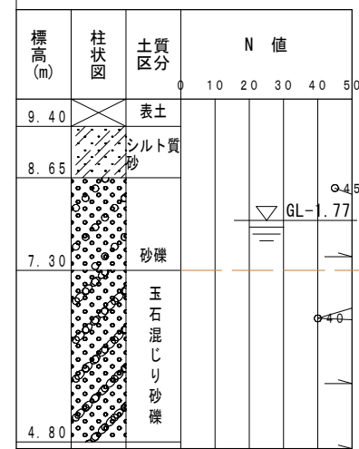
推定土質柱状図
