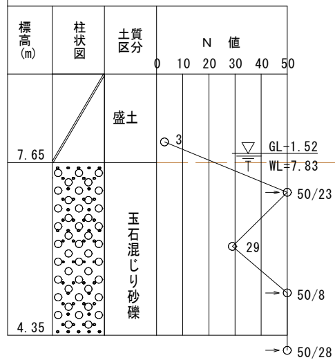
推定土質柱状図
